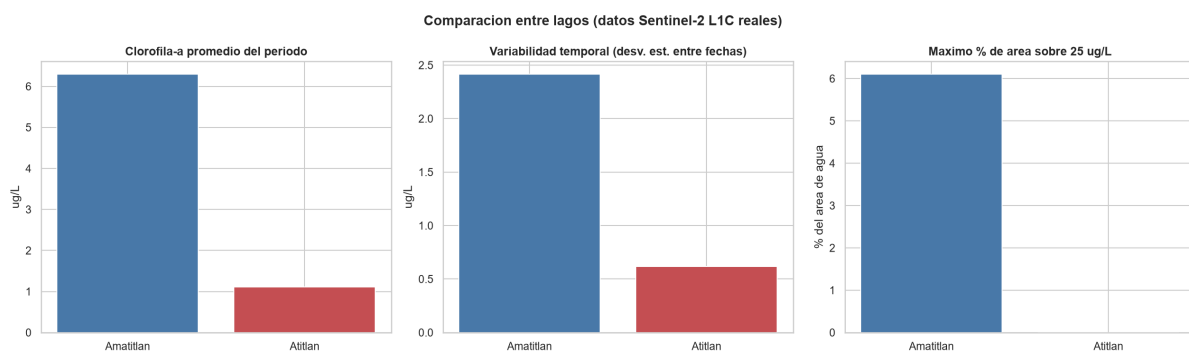
Comparación entre lagos: concentración promedio, variabilidad y superficie afectada.
