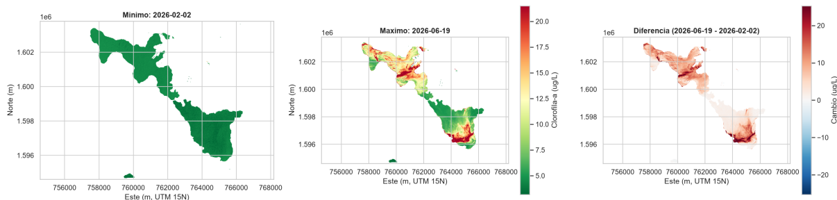
Lago de Amatitlán: comparación entre su mejor y su peor fecha, y mapa de cuánto cambió cada zona.
