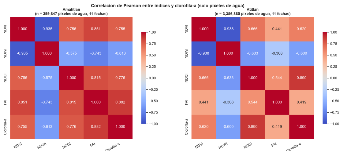
Relación entre los índices calculados y la clorofila-a, en cada lago.
