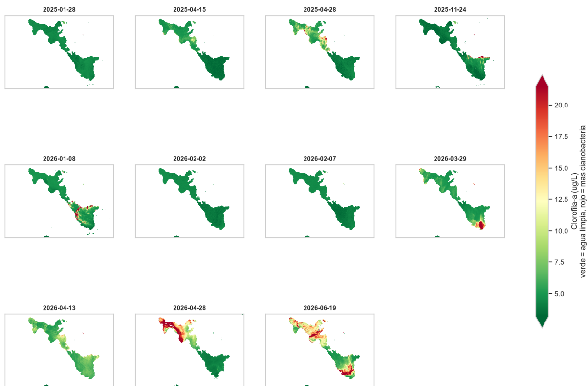
Lago de Amatitlán: clorofila-a en las 11 fechas, misma escala de color.
