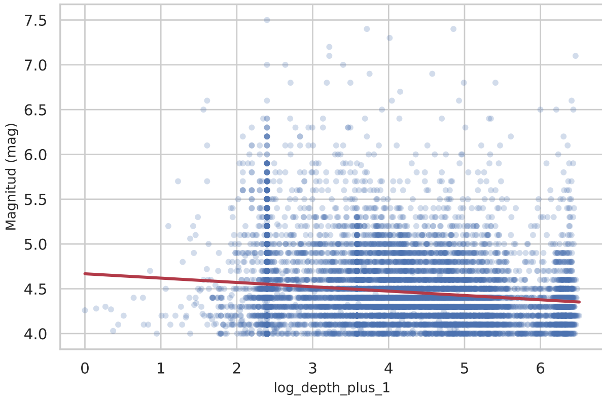
Magnitud vs \log(\text{profundidad} + 1)
