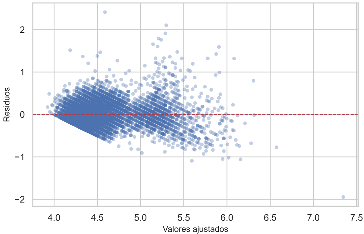
Residuos vs ajustados (M4)
