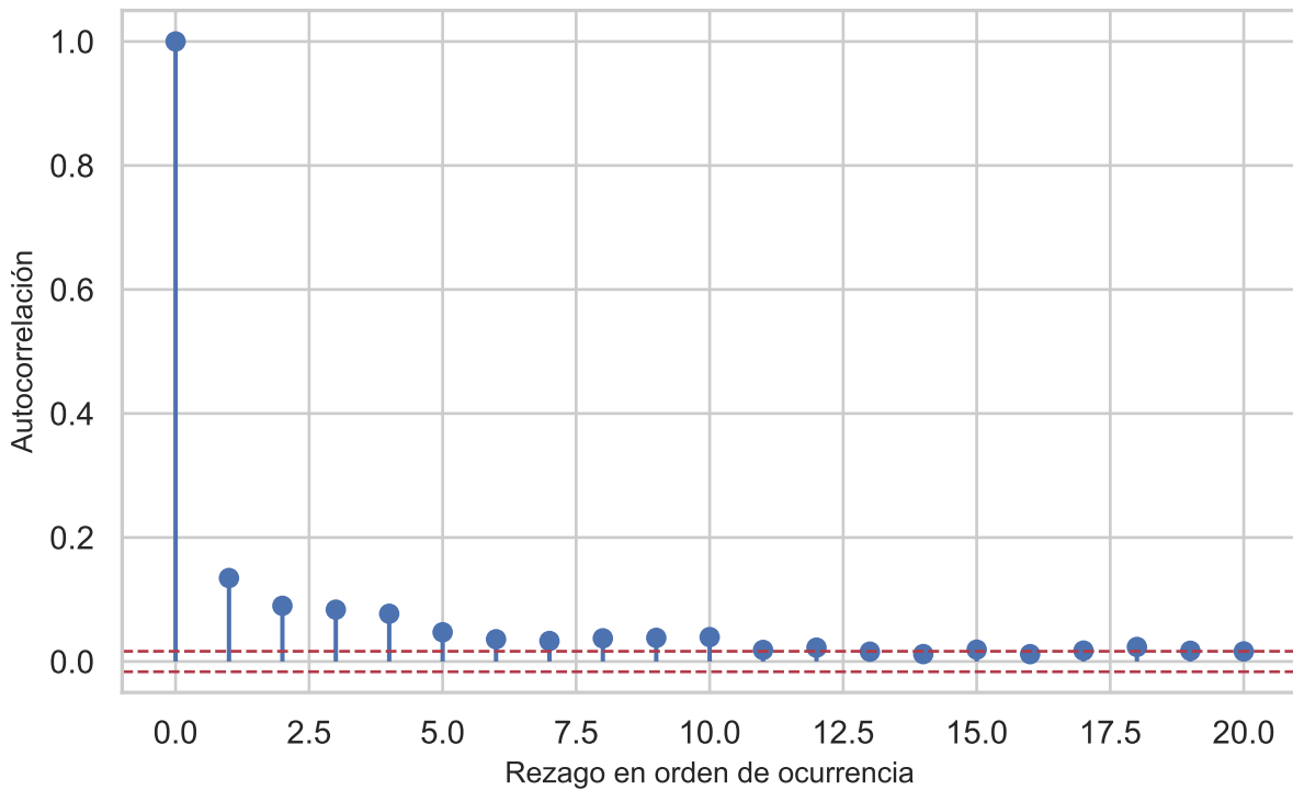
Modelo final: ACF de residuos ordenados por tiempo
