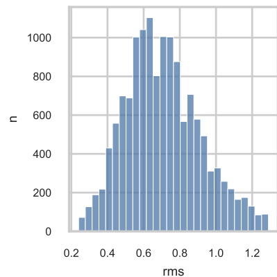
rms (p1-p99)
