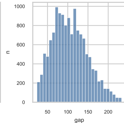
gap (p1-p99)
