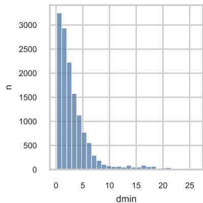
dmin (p1-p99)
