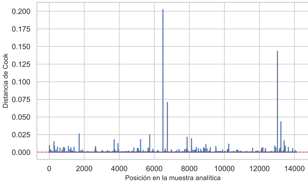
Modelo final: distancia de Cook
