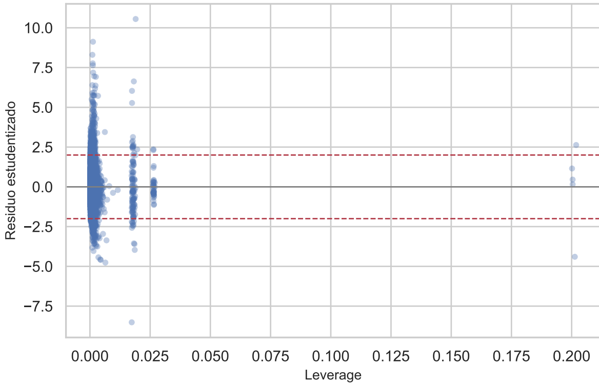
Leverage vs residuos estudentizados (M4)
