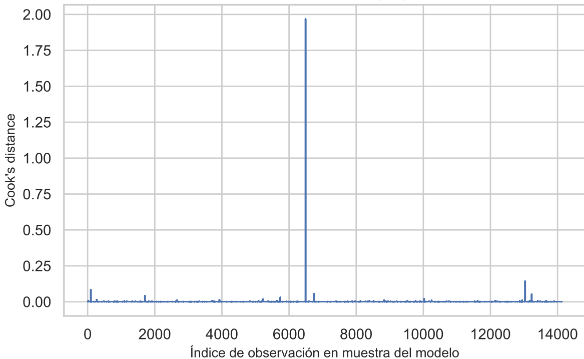
Distancia de Cook (M4)
