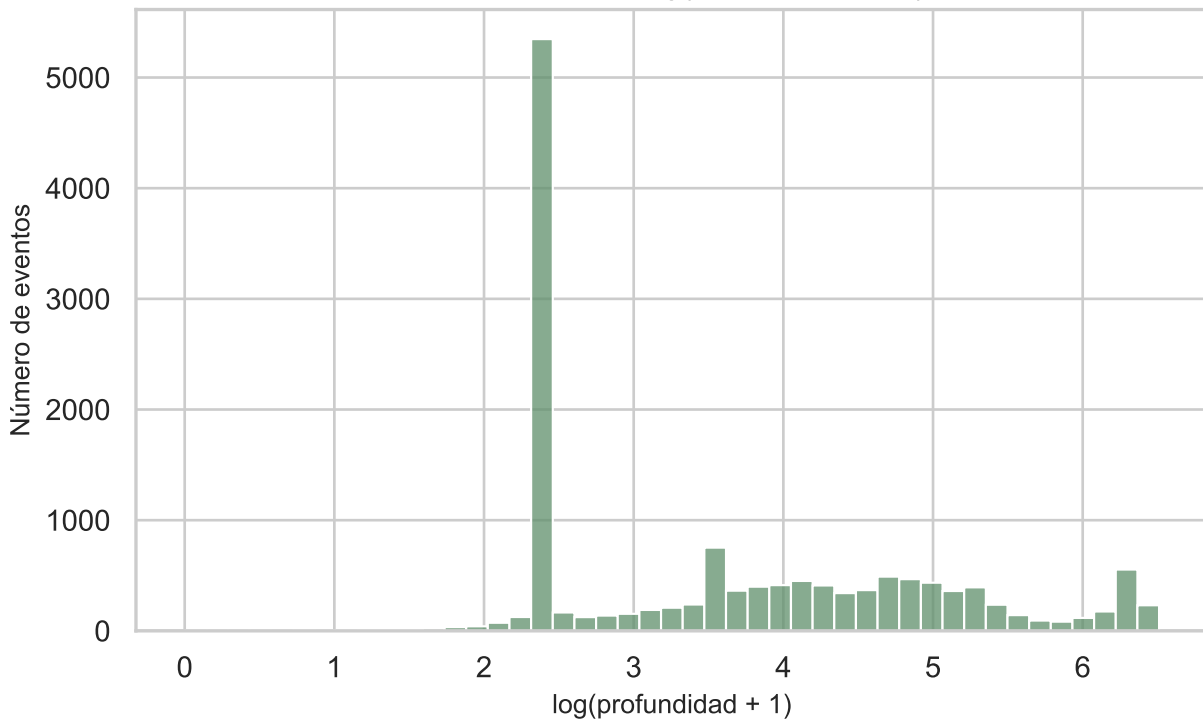
Distribución de \log(\text{profundidad} + 1)
