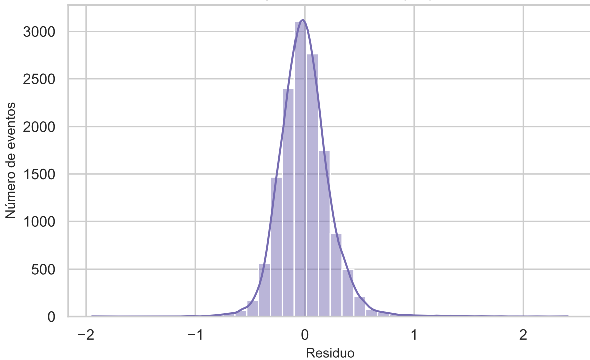
Histograma de residuos (M4)
