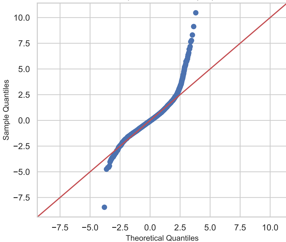
QQ-plot de residuos (M4)
