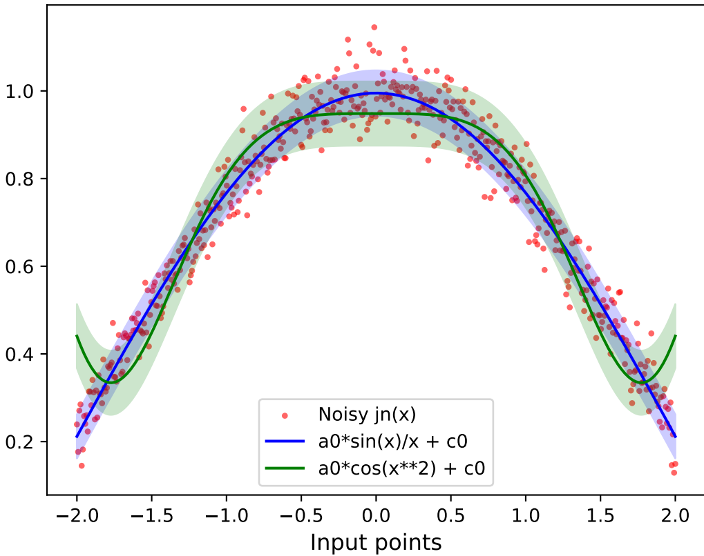
SISSO Functions
