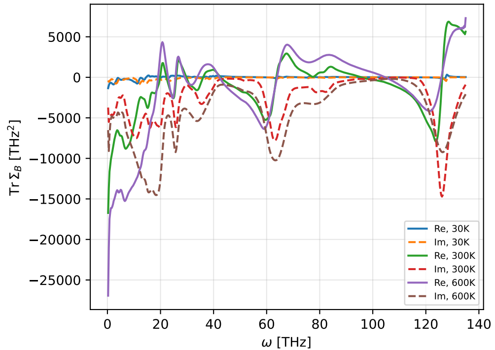
d5a: bubble \text{Tr } \Sigma_B(\omega)
