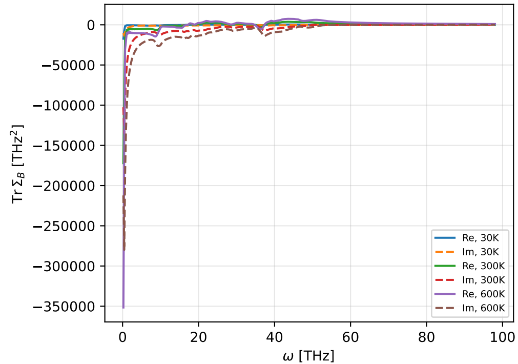
cnt33: bubble \text{Tr } \Sigma_B(\omega)
