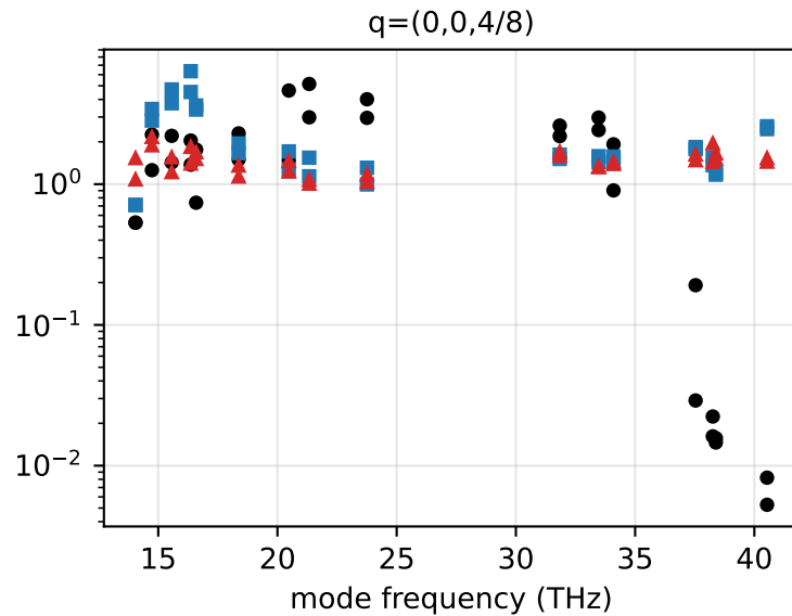
CNT(3,3) 3-phonon linewidths, conserving vertex (mesh 8, eta 0.2, T=300K)
