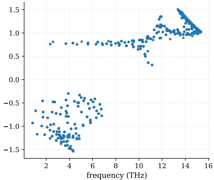
mode Grueneisen \gamma
