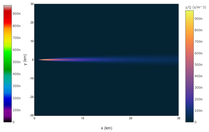
(b) Diluție atmosferică, hartă termografică
