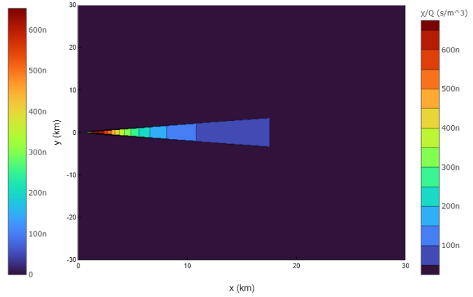
(b) Diluție atmosferică, reprezentare tip contur
