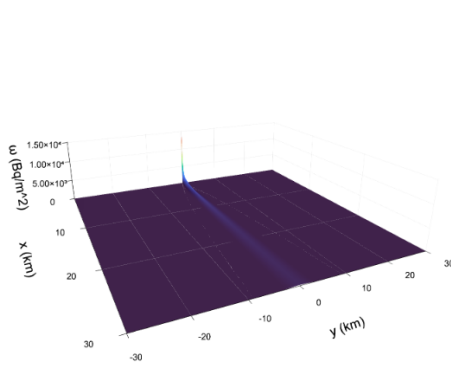
(c) Depuneri pe sol, suprafață 3D
