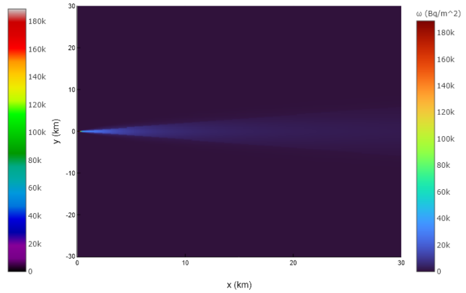
(d) Depuneri pe sol, hartă termografică
