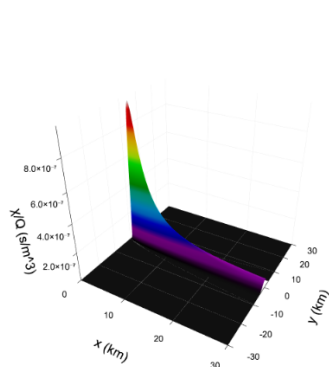
(a) Diluție atmosferică, suprafață 3D
