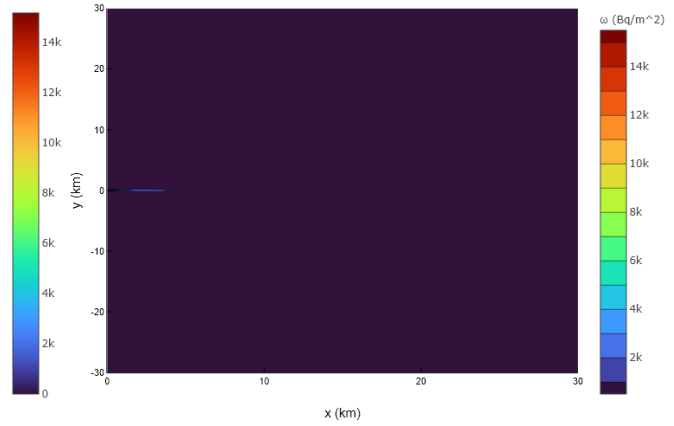
(d) Depuneri pe sol, reprezentare tip contur
