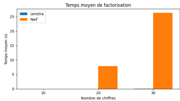
Fig. 4. – Comparaison des algorithmes naïfs et de Lenstra pour des nombres tirés aléatoirement
