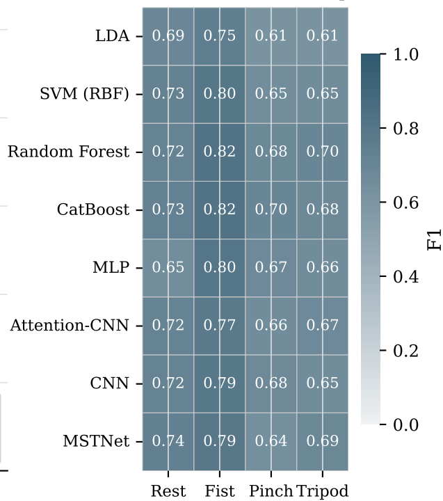
Per-Class F1 Heatmap
