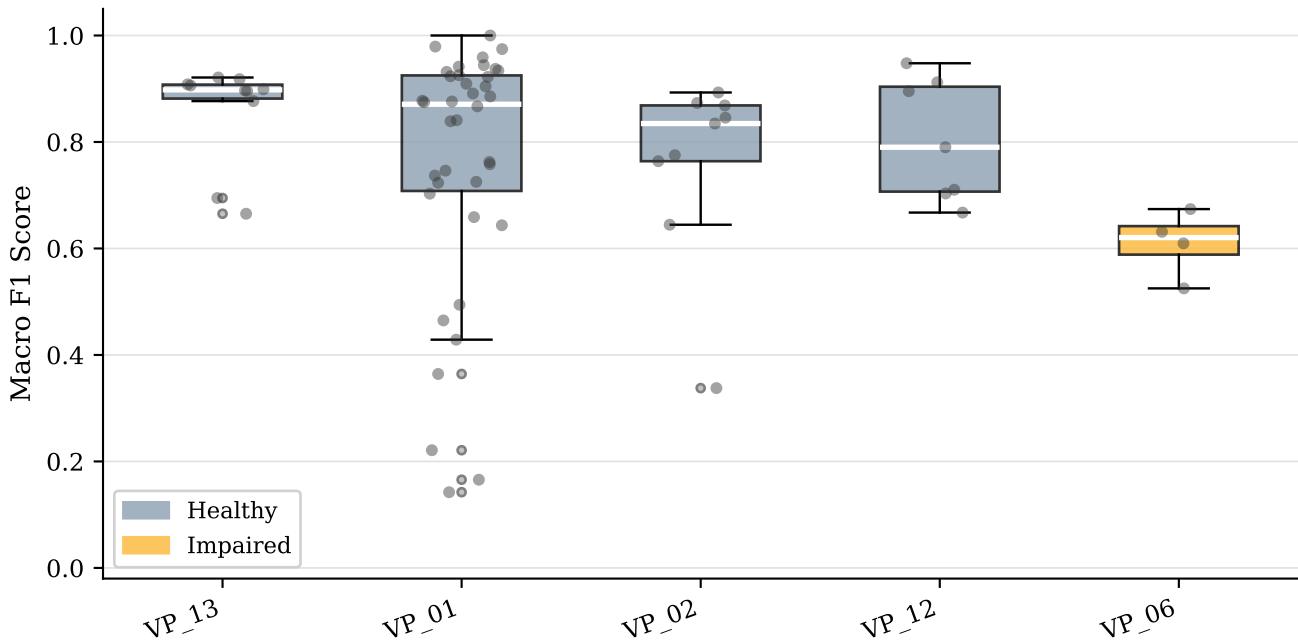
Per-Fold F1 Distribution per Participant — CatBoost
