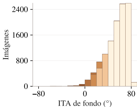
(d) PAD-UFES-20
