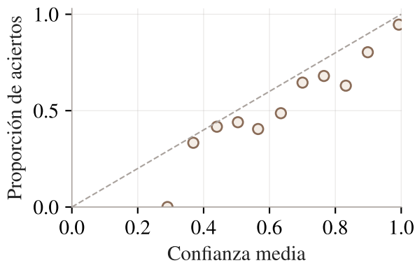
(a) Público · protocolo B71 ECE = 0,0688
