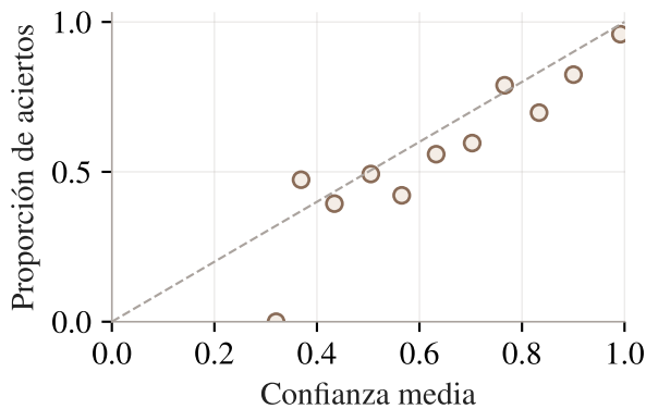
(e) B71 ECE = 0,0529
