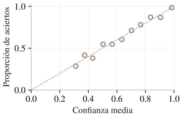
(c) A71 ECE = 0,0154
