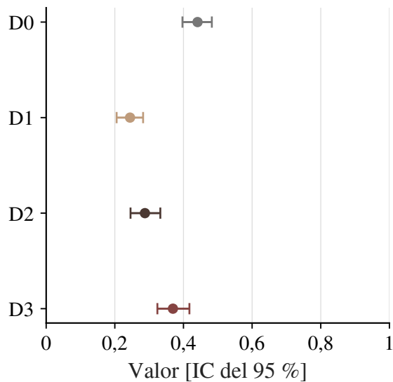
F1 macro
