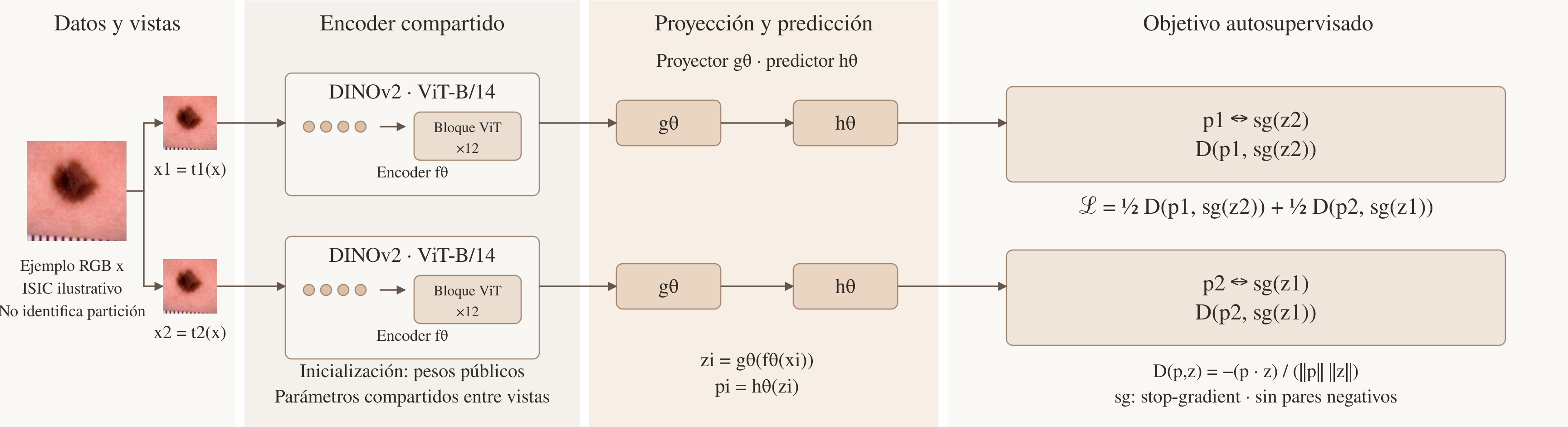
(a) Entrenamiento SimSiam (D2 / D3)
