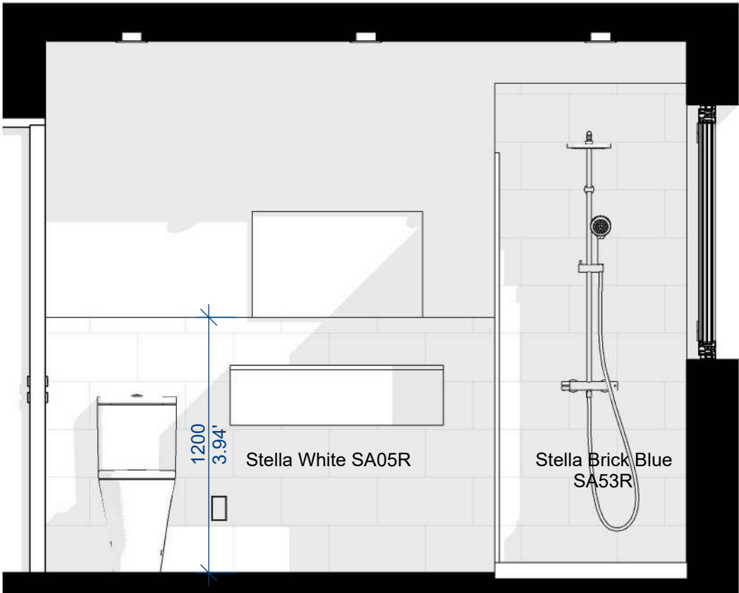
3 Section A 1 : 25
