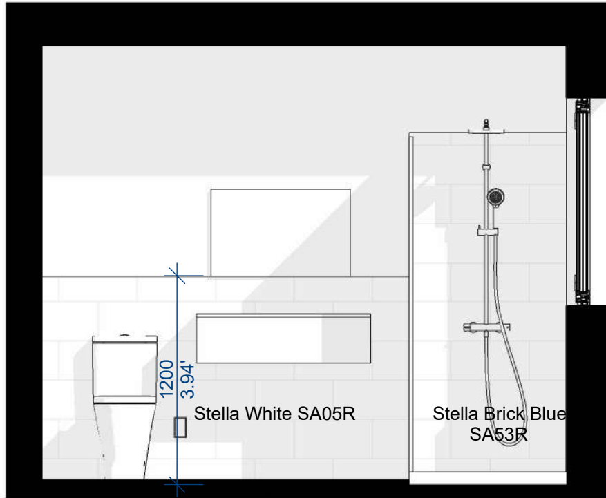
3 Section B' 1 : 30
