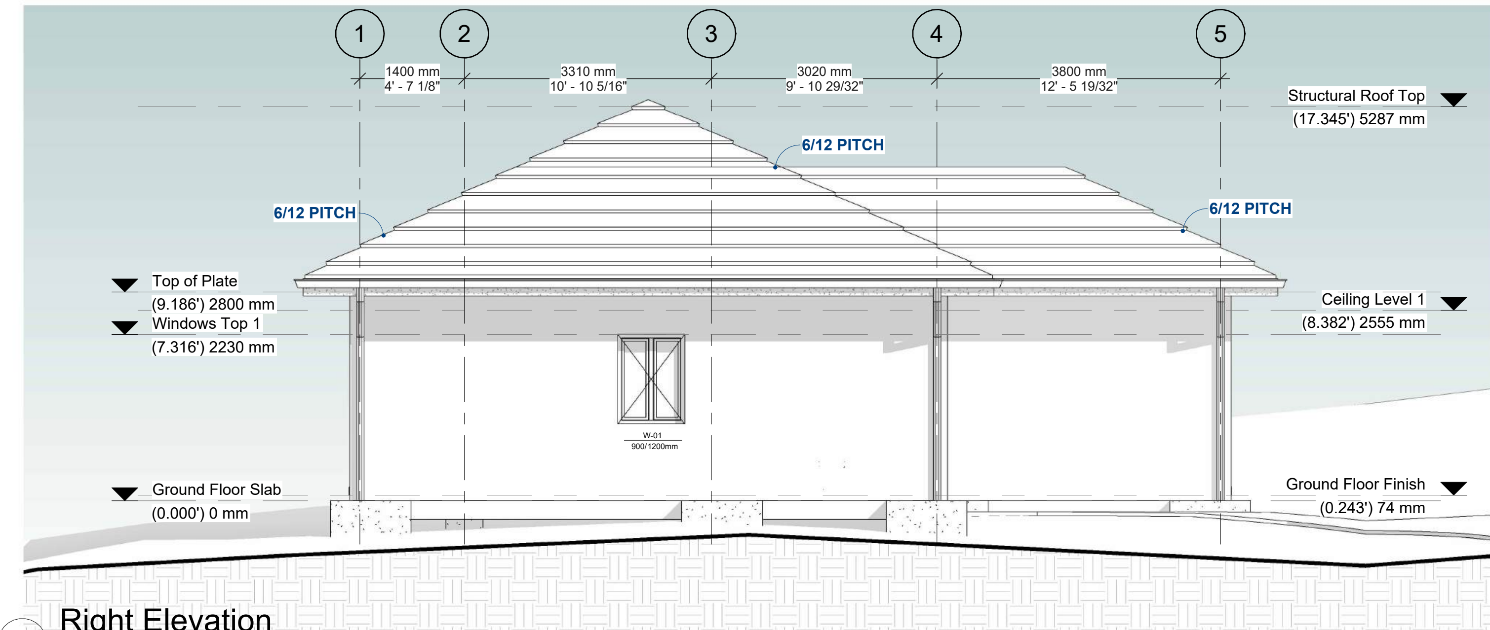
2 Right Elevation 1 : 50
