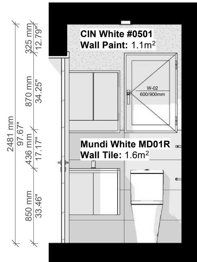
1 Section A' 1 : 25
