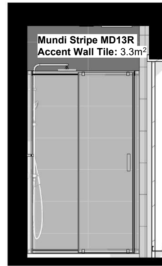
2 Section B' 1 : 25
