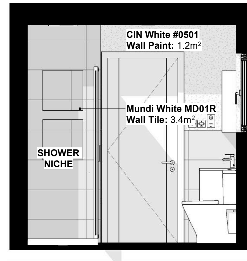
7 Section D' 1 : 25
