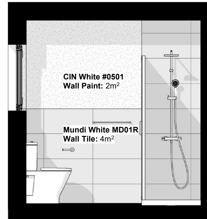
3 Section C' 1 : 25
