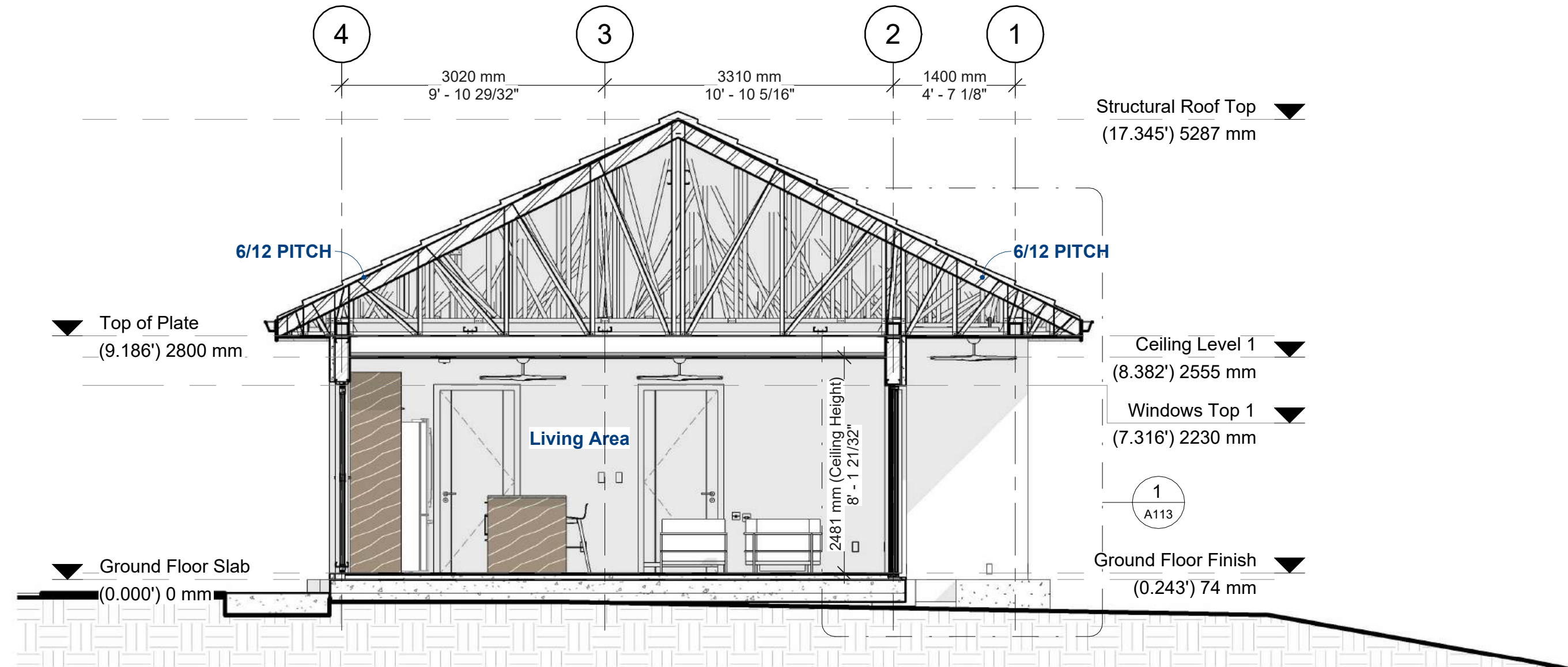
Section 3 1 : 50
