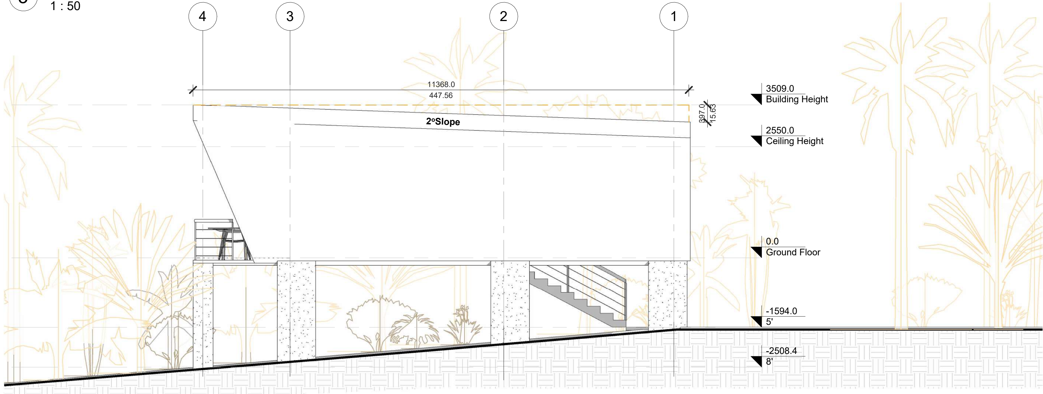
2 Right Elevation 1 : 50
