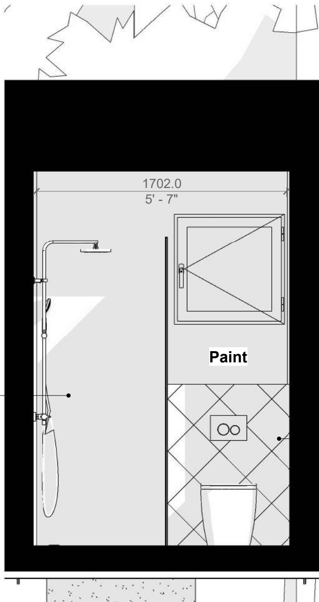
1 Section 7 1 : 25
