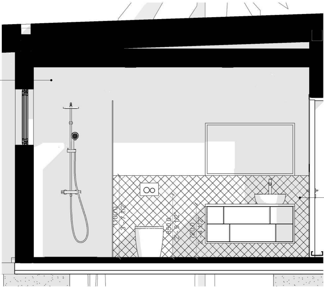
1 Section 6 1 : 25
