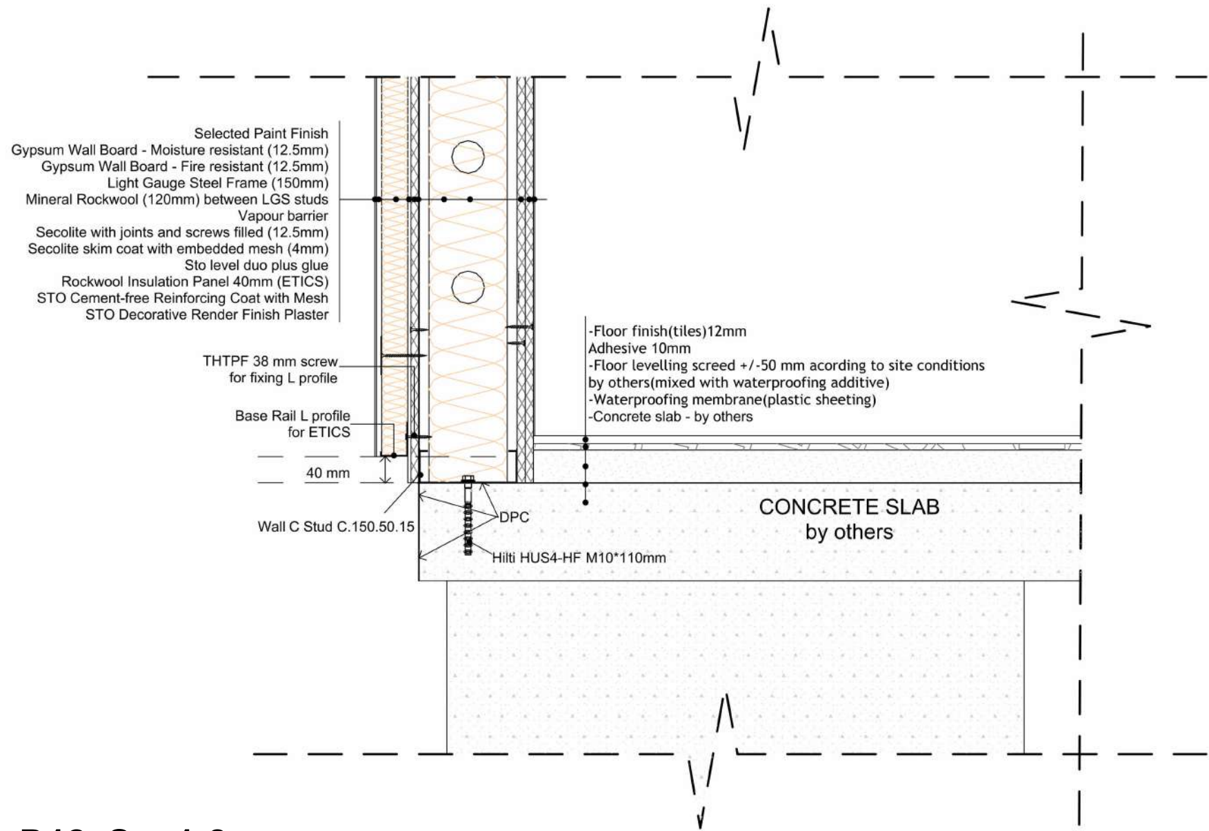
D12. Sc: 1:8
