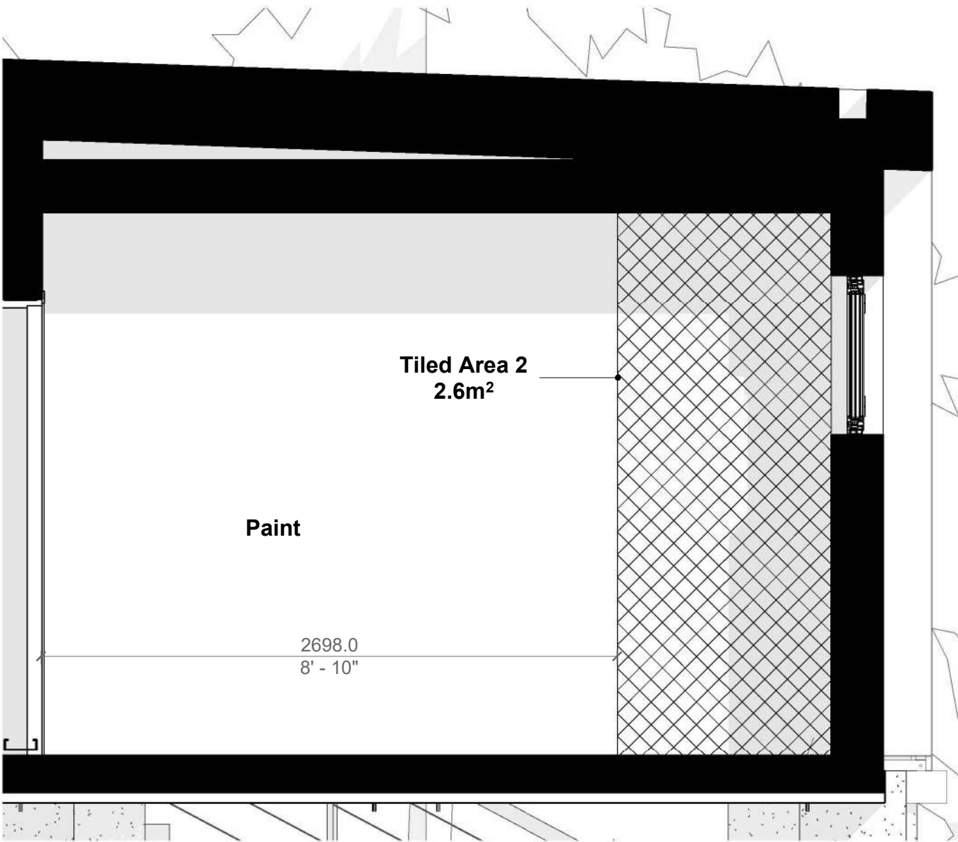
4 Section 12 1 : 25
