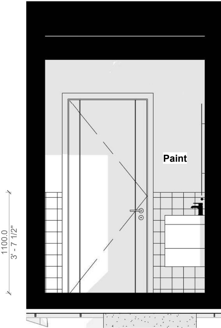
3 Section 9 1 : 25
