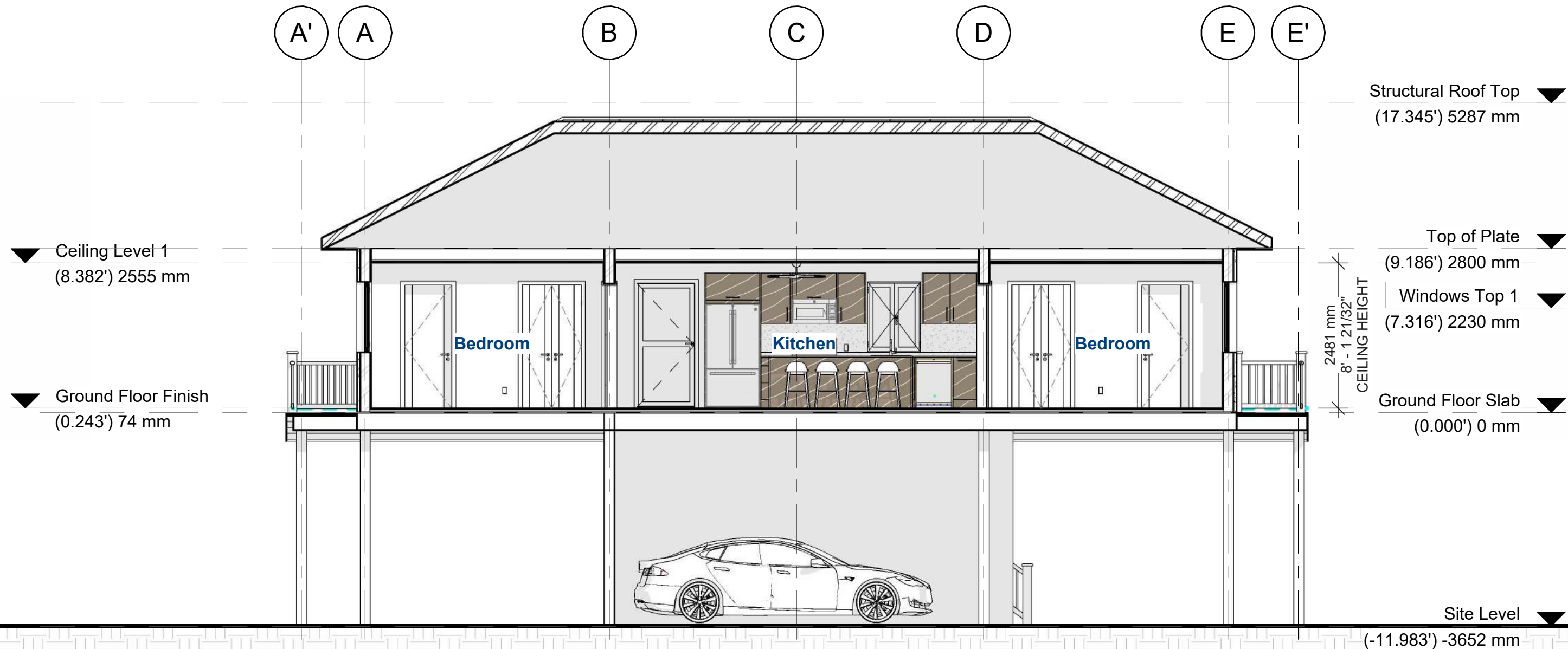
2 Section 2 1 : 70
