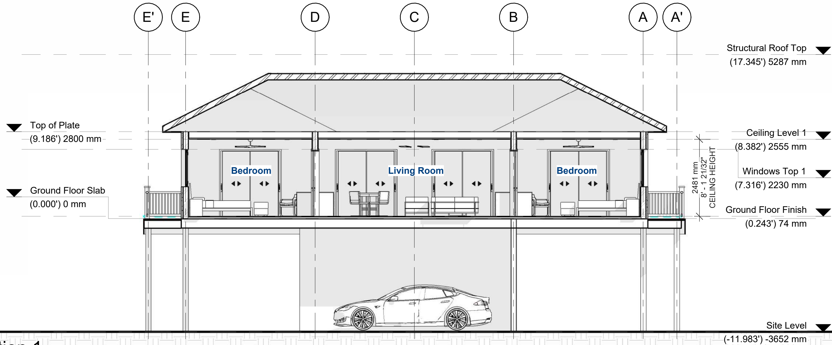
1 Section 1 1 : 70
