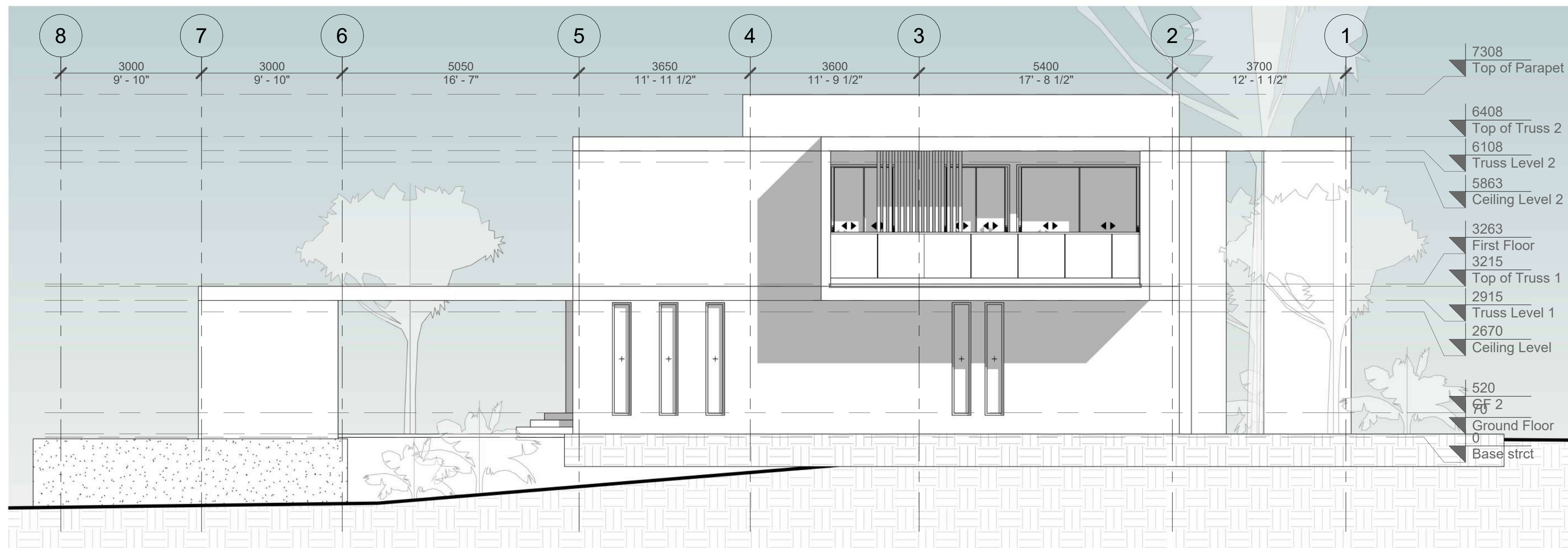
1 Right Elevation
