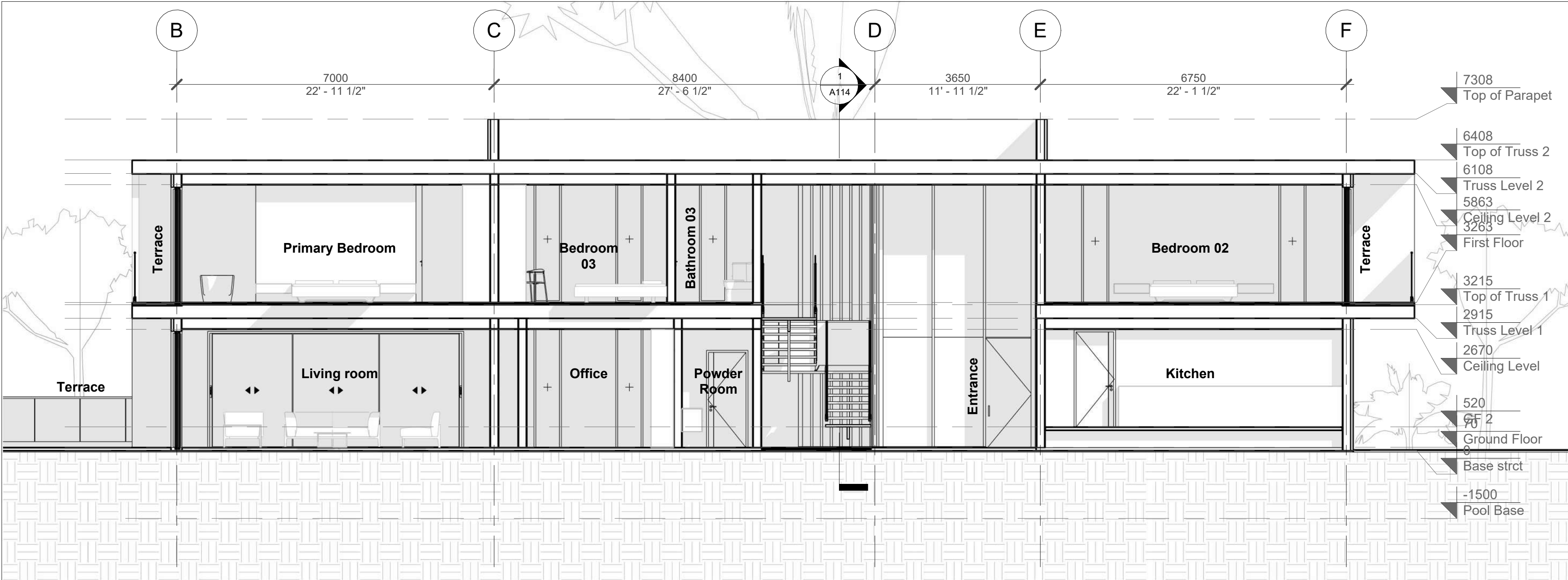
Section 2 1 : 70
