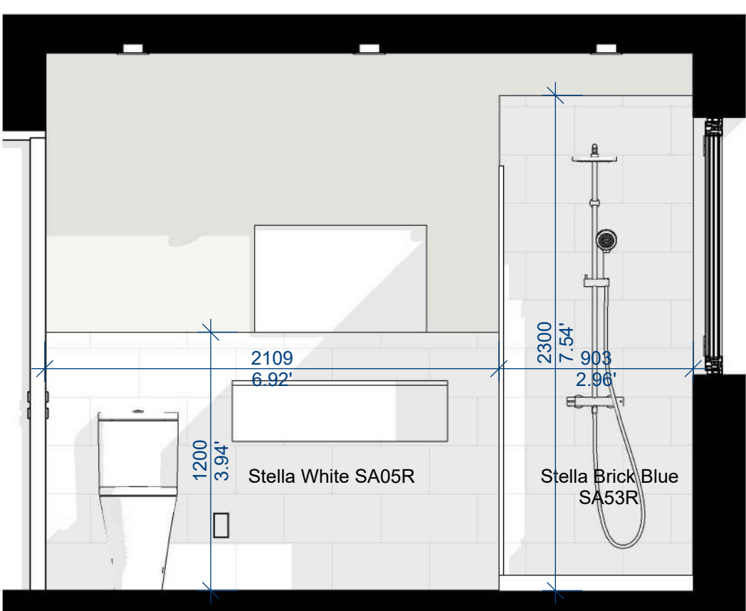
3 Section A 1 : 25
