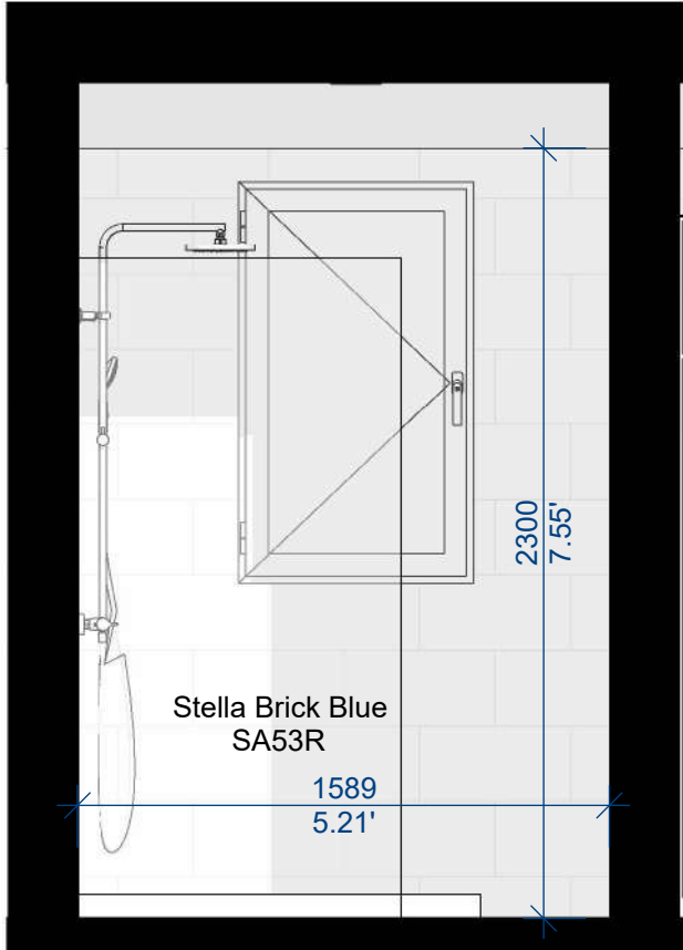
5 Section C 1 : 25
