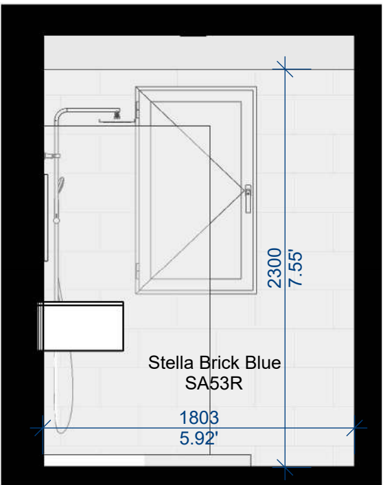
2 Section A' 1 : 30
