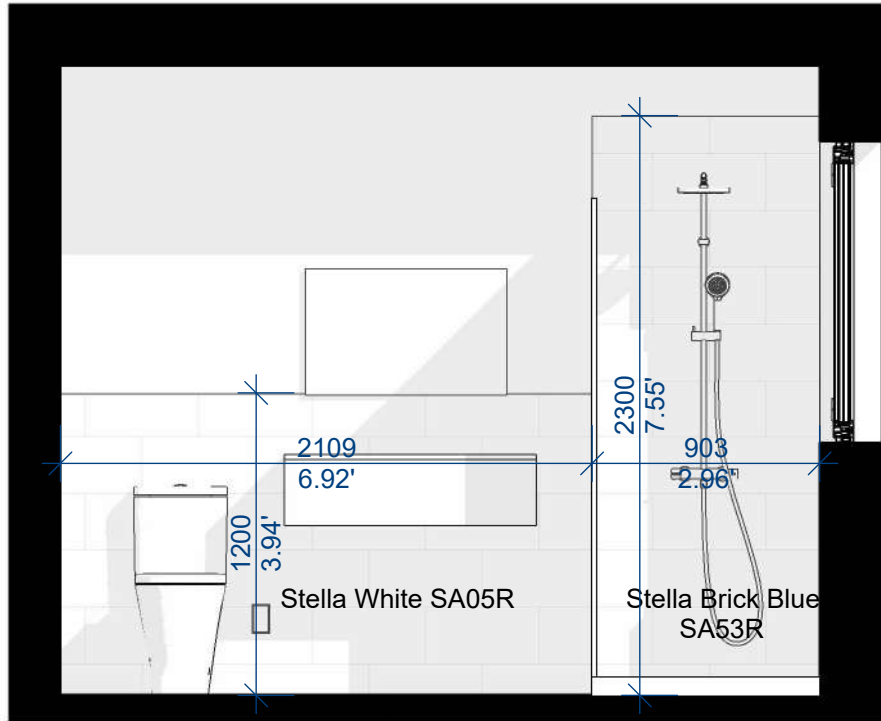
3 Section B' 1 : 30
