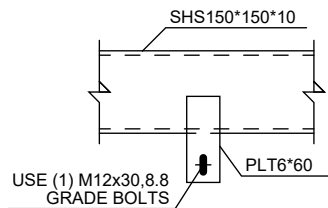
A - A
