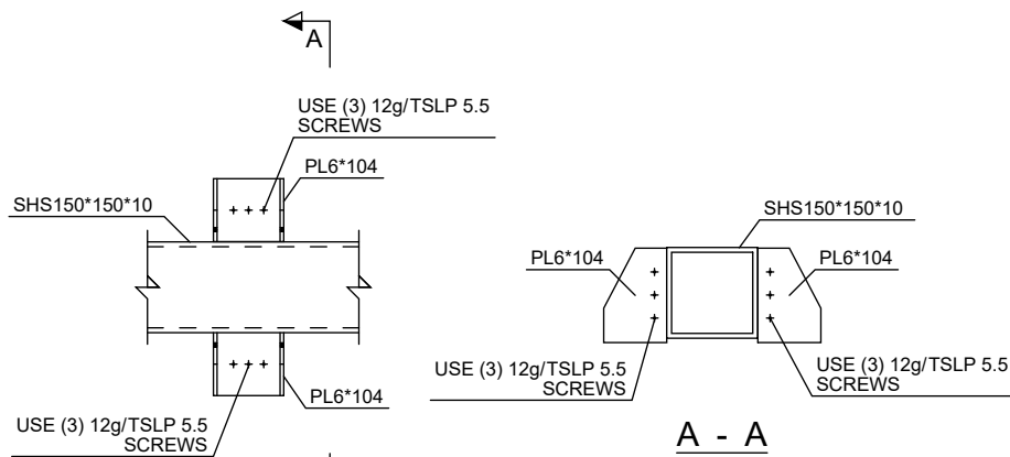
A - A
