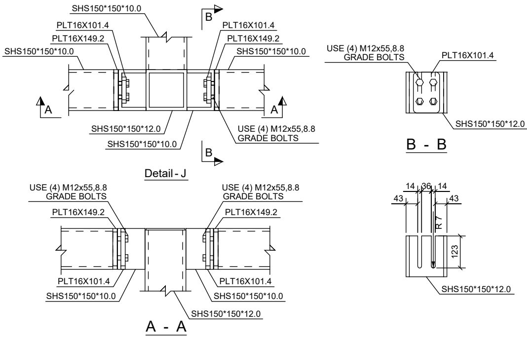
A - A
