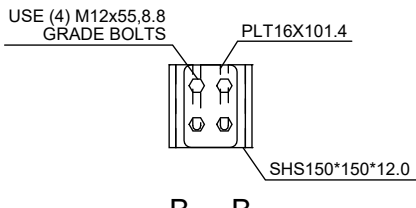
B - B
