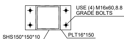
B - B
