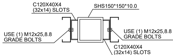
A - A
