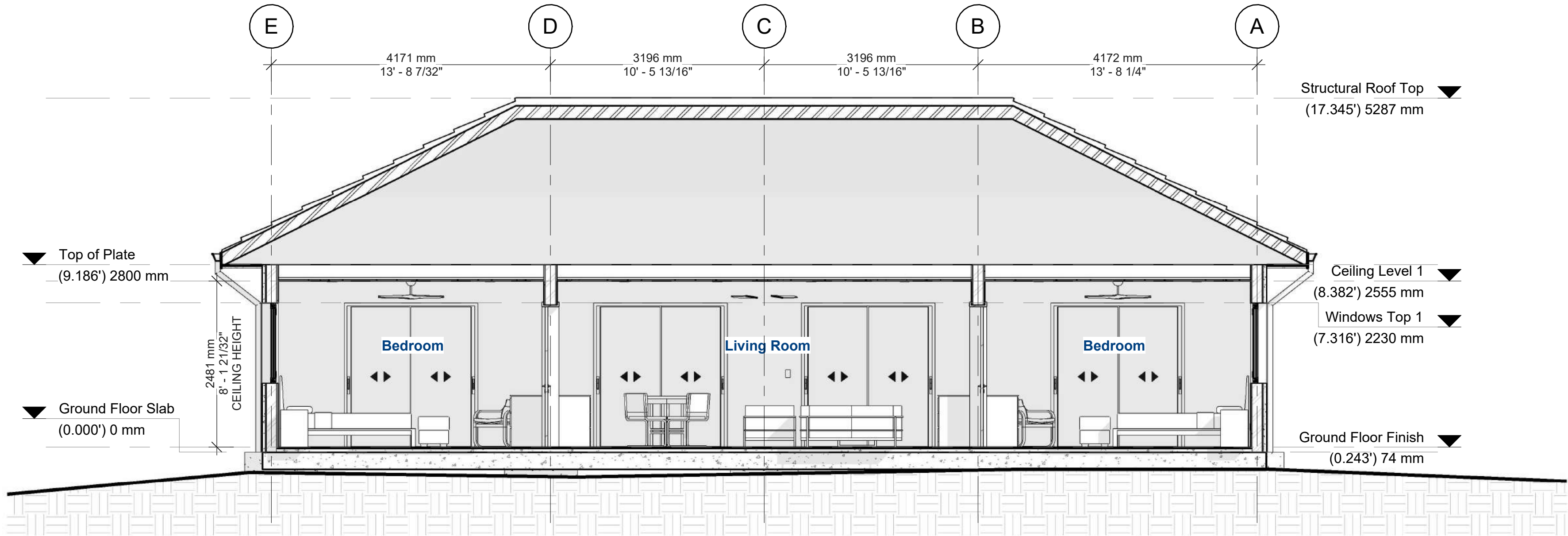
Section 1 1 : 50
