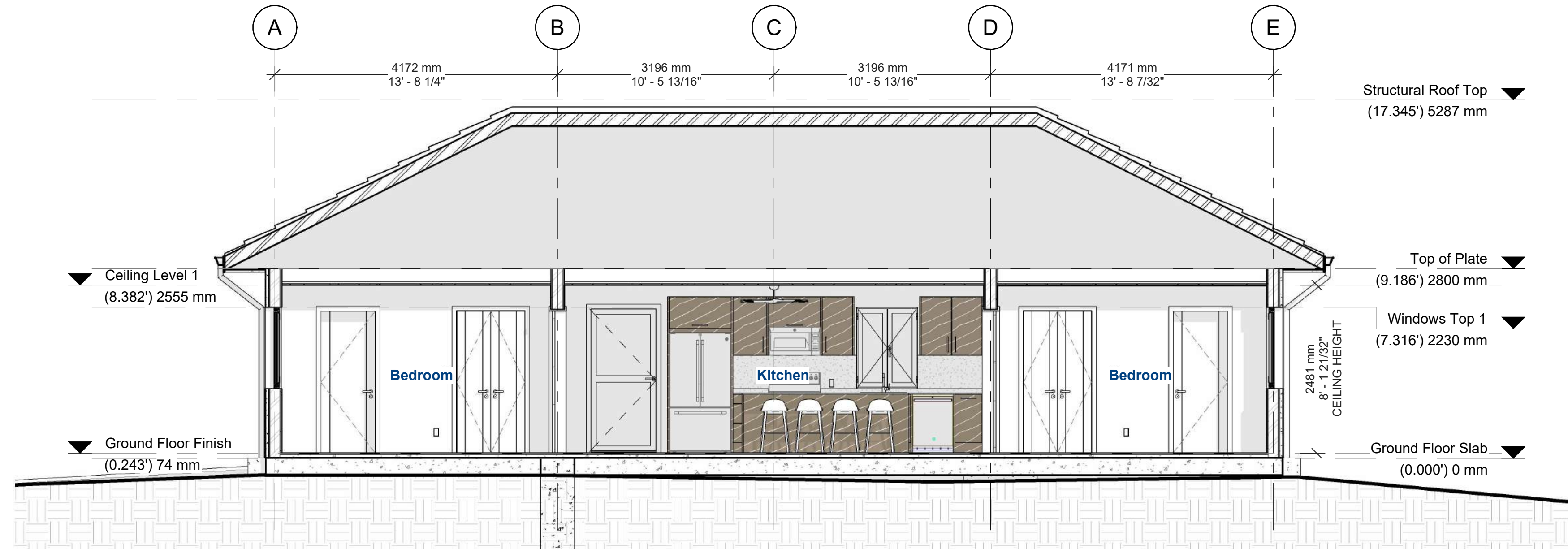
Section 2 1 : 50
