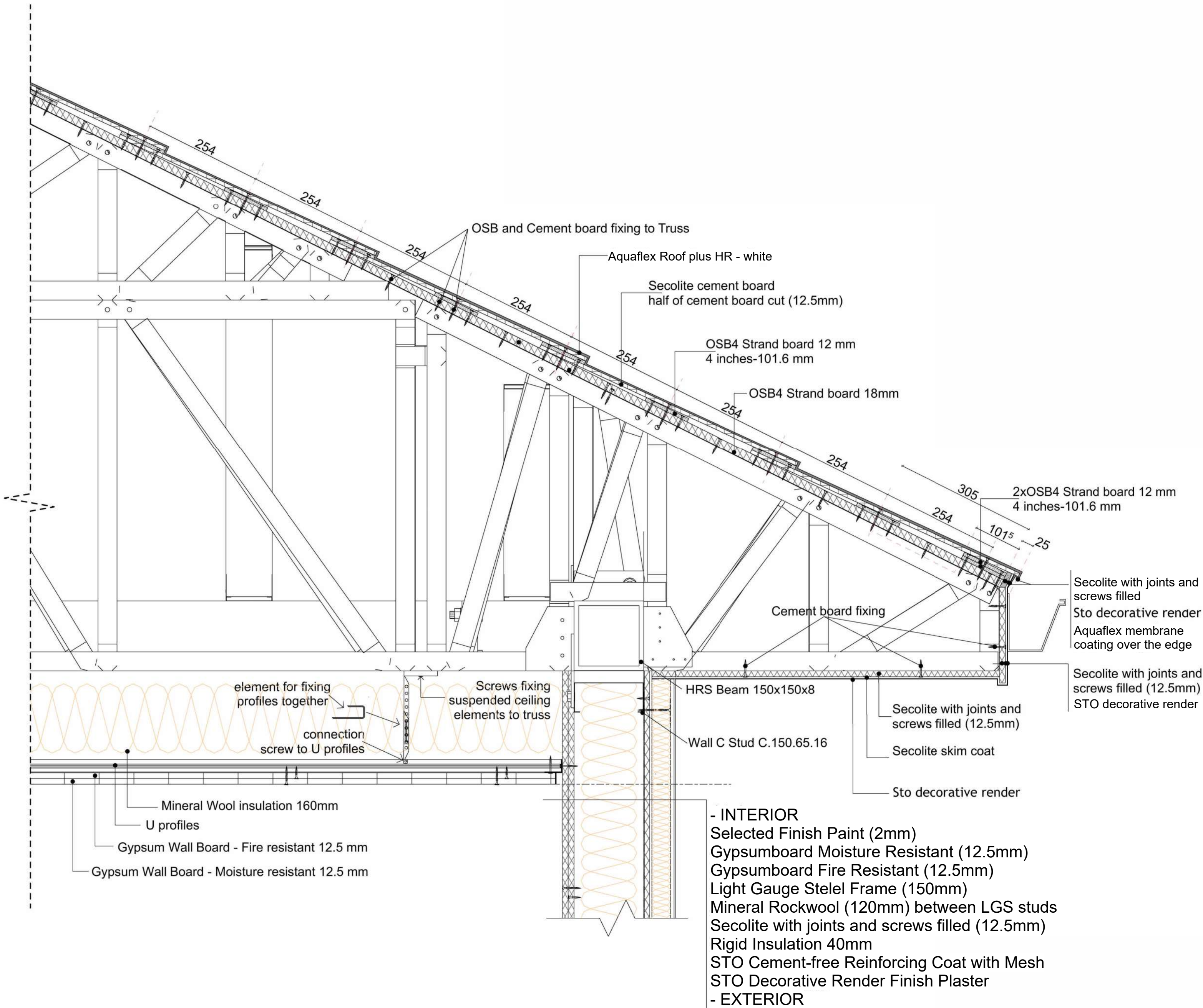
D11.Island Style Roof Detail
