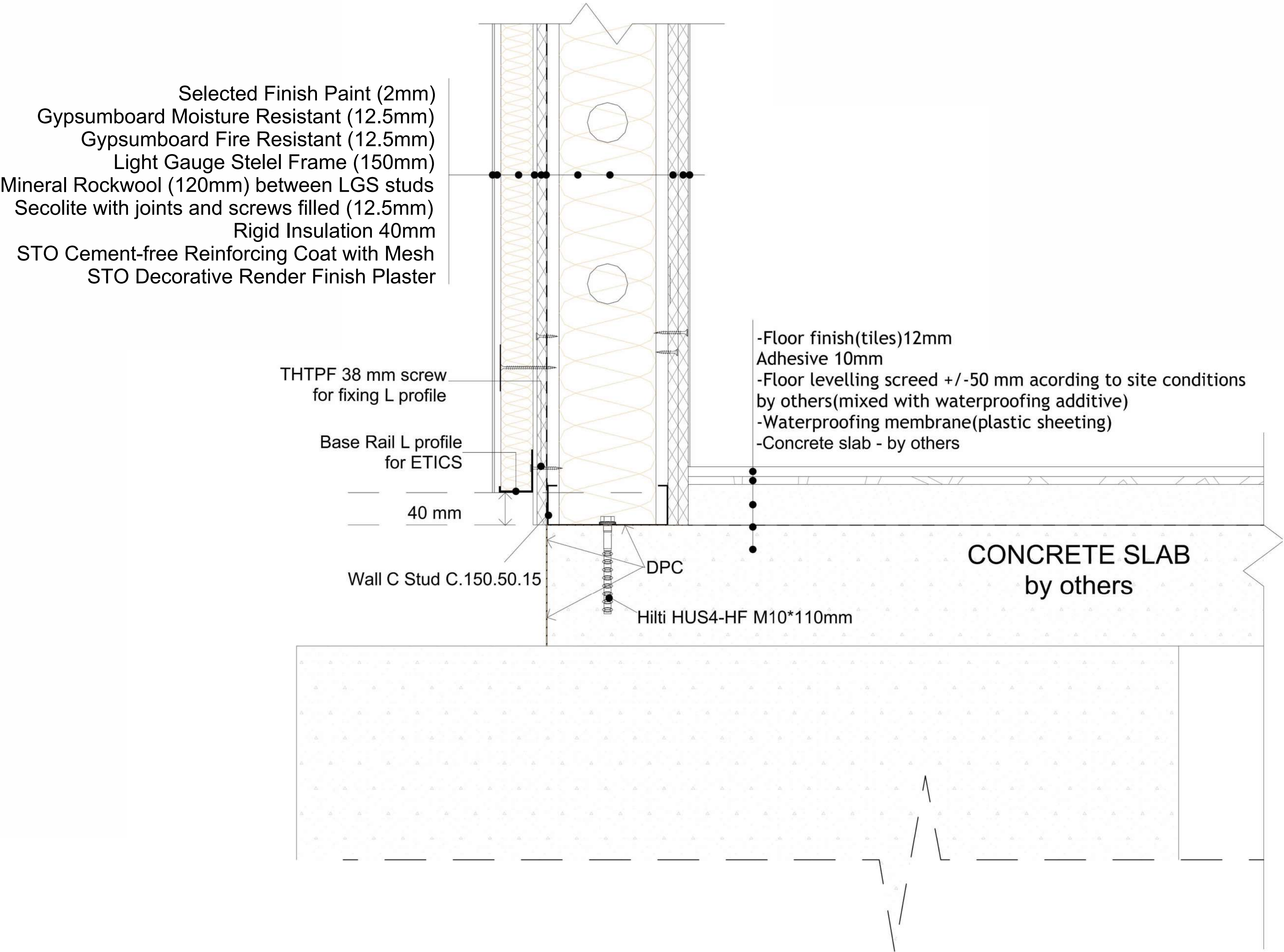
D14.Exterior wall base Detail
