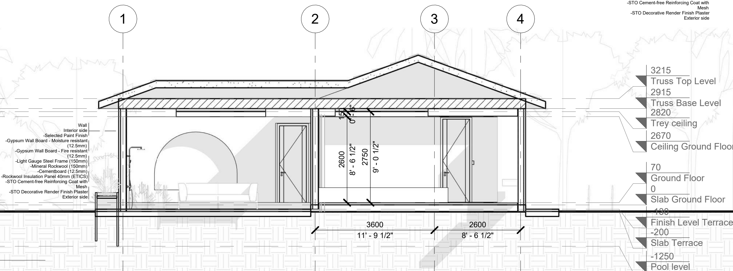
3 Section 3 1 : 65
