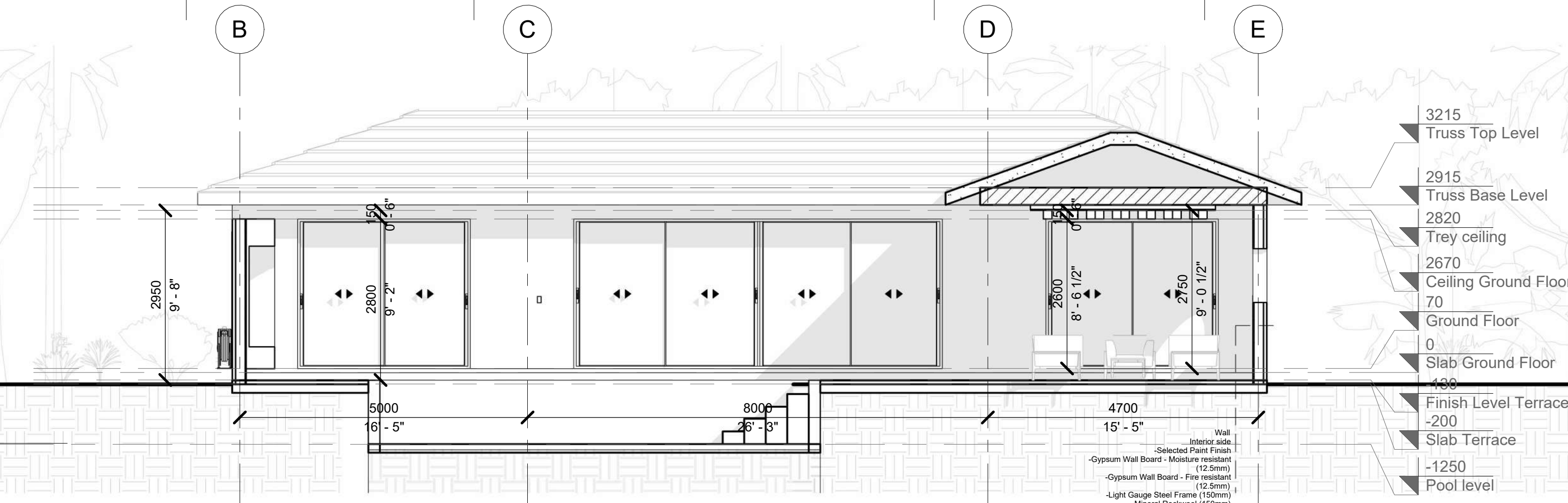
2 Section 2 1 : 65
