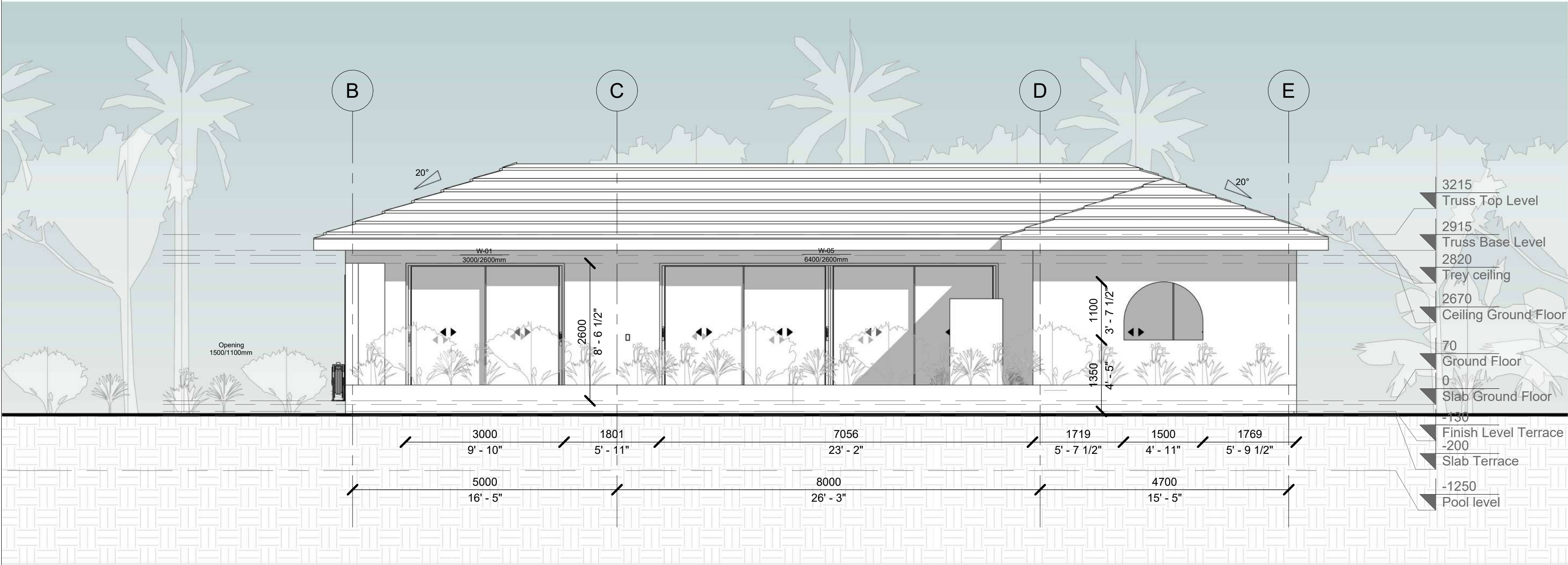
2 Back Elevation 1 : 60
