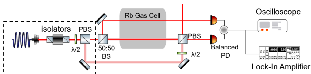
圖(二)雷射保護與幫浦光、探測光分配之光路圖
