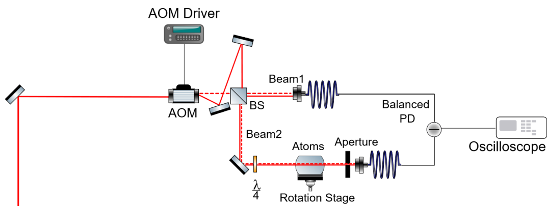
圖(十二)馬赫—曾德爾干涉儀完整光路配置圖
