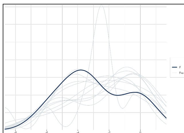
5b) Posterior predictive check
