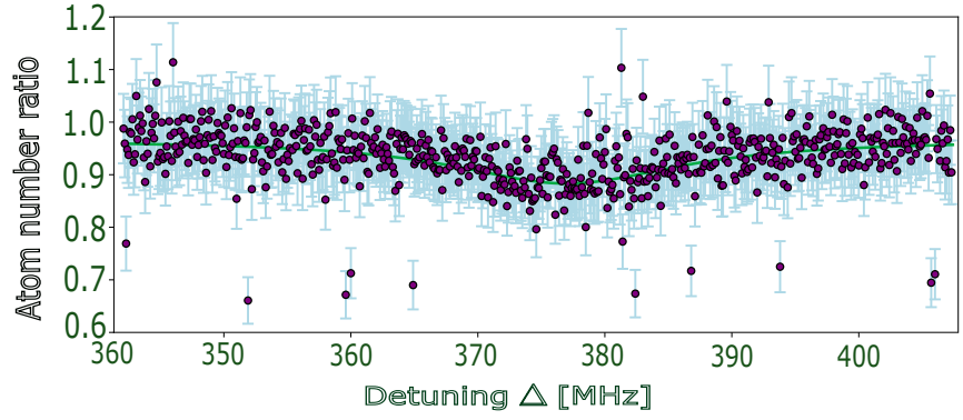
(a) attention premier trait 360 au lieu de 340 Resonance spectrum at 375.74 \pm 0.48 MHz ( I = 5.6 W/cm 2 for t = 1000 ms).
