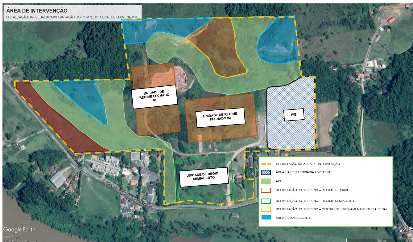
Figura 8 - Área de intervenção do Complexo Prisional
