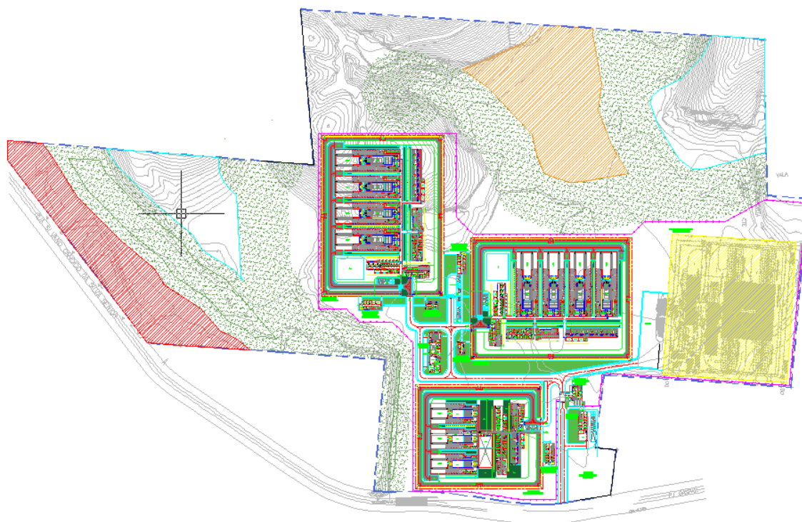
Figura 9 - Implantação do Complexo Prisional
