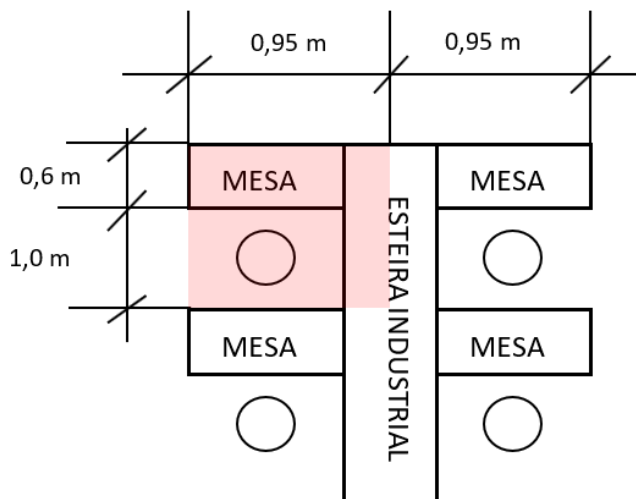
Figura 12 - Simulação da Área de trabalho para artigos de iluminação
