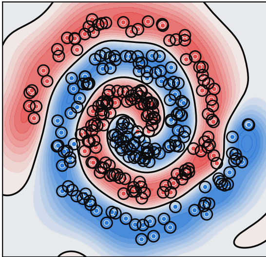
LSSVM-Std (denso) (0% esparso)
