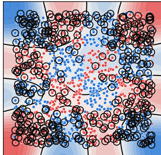
(70% esparso)
