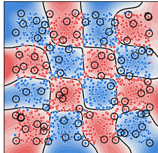
(94% esparso)
