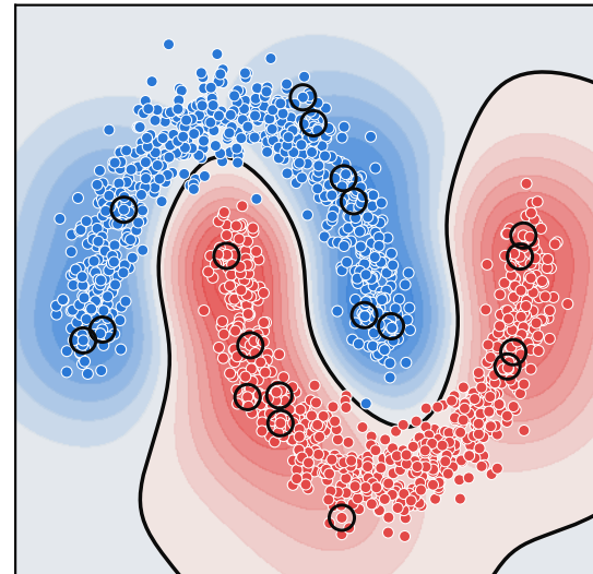
(99% esparso)
