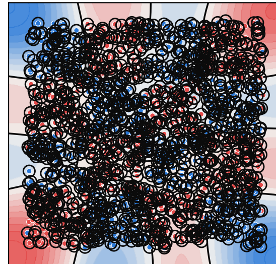
(2% esparso)
