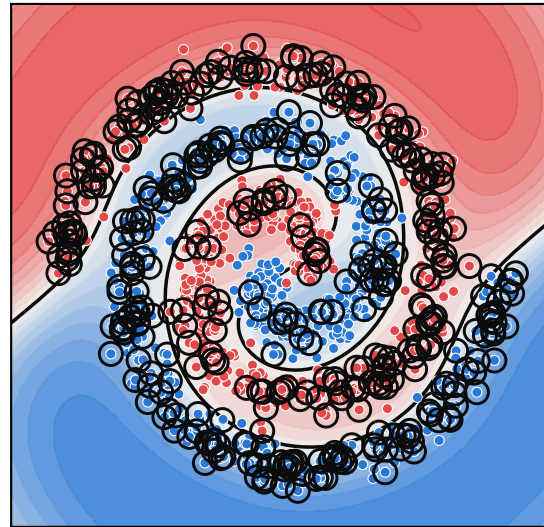
Nyström-SVM (70% esparso)
