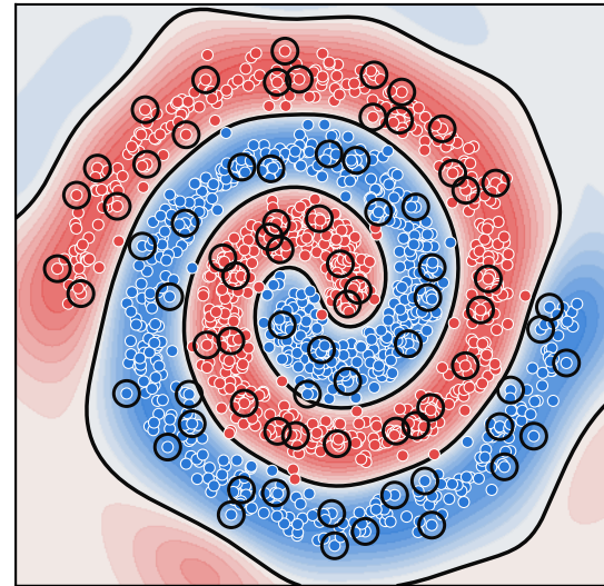
ADMM-Nyström (94% esparso)
