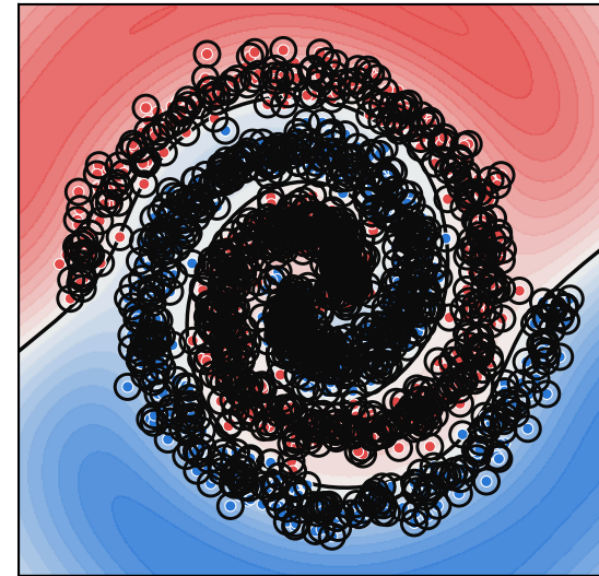
DualFISTA (4% esparso)
