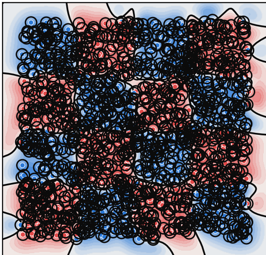
(0% esparso)
