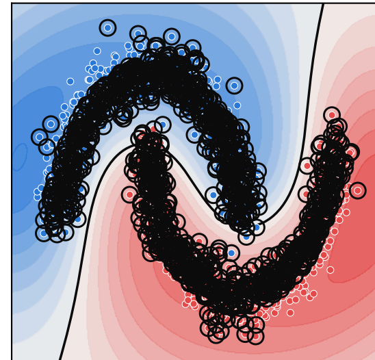
(19% esparso)
