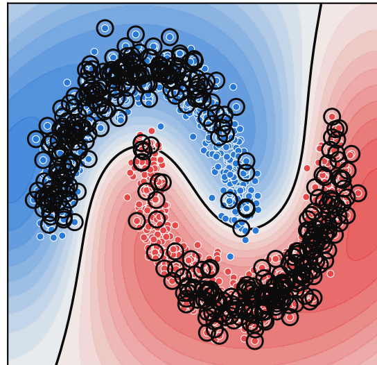
(70% esparso)
