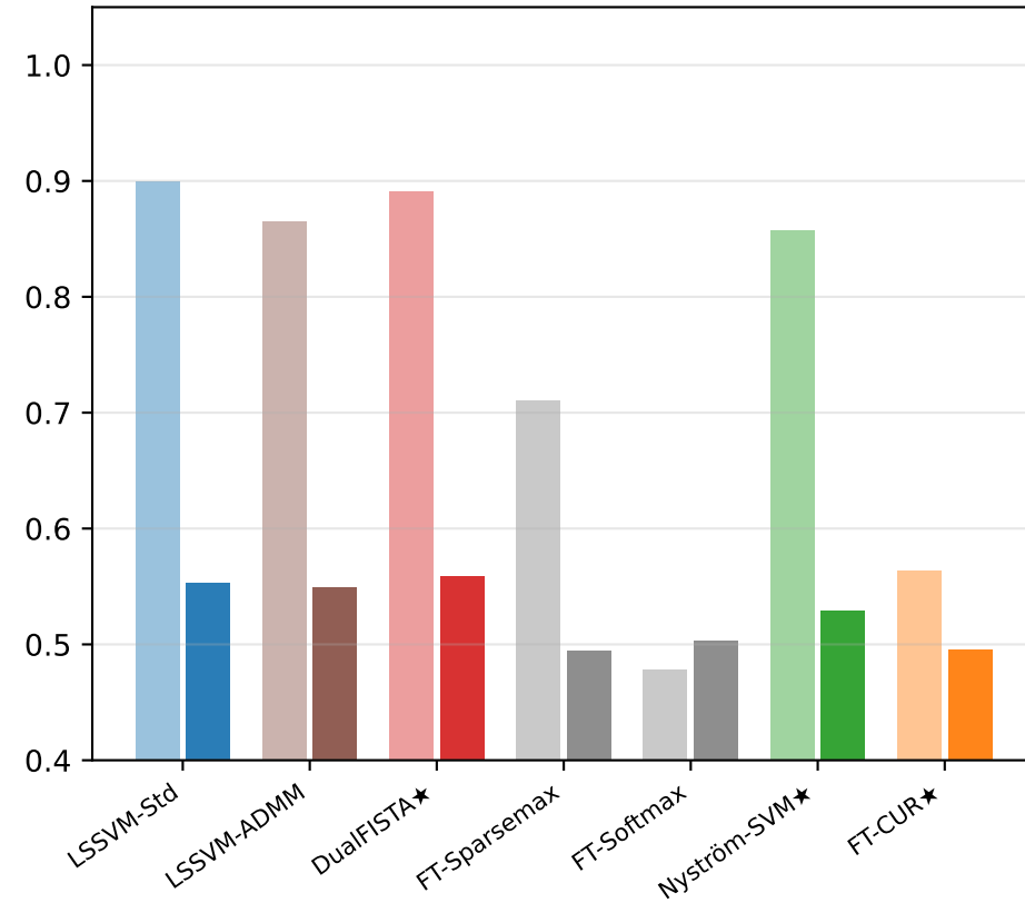
Dataset: TWC
