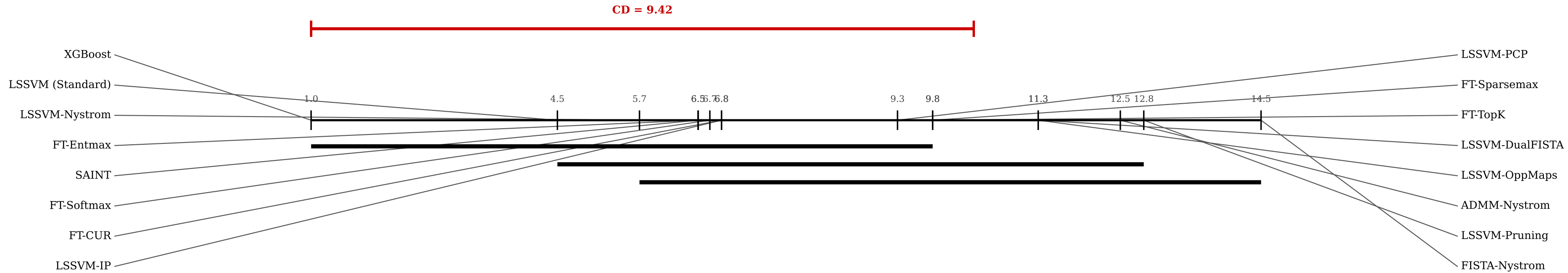
Diagrama de Diferença Crítica — F1-macro (Tier 2)
