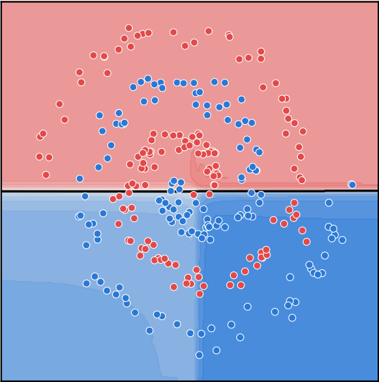
SAINT (inter-instâncias)
