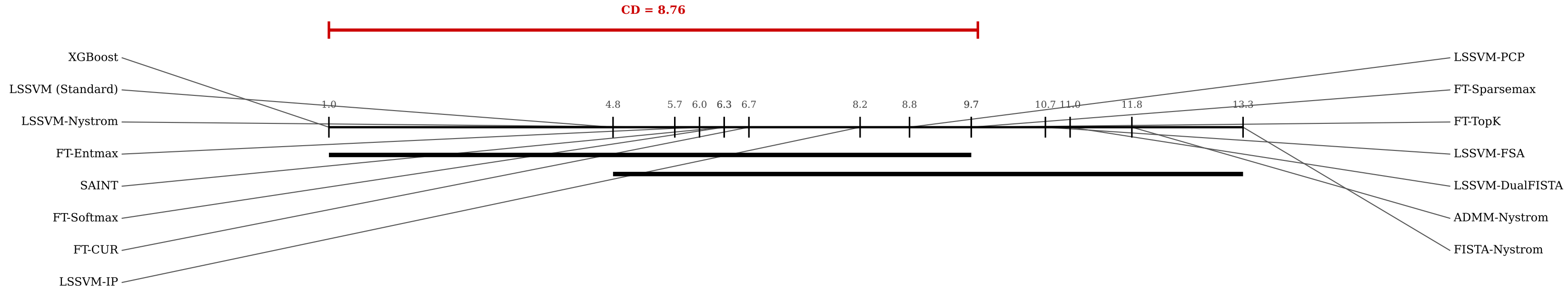
Diagrama de Diferença Crítica — F1-macro (Tier 2)
