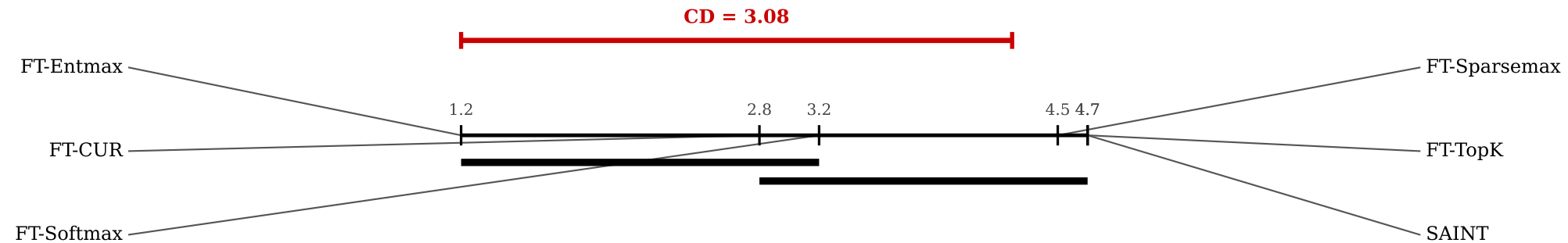
Diagrama de Diferença Crítica — F1-macro (Tier 2 — Transformers)
