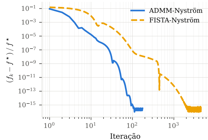
(a) Sub-otimalidade — cada solver no seu objetivo
