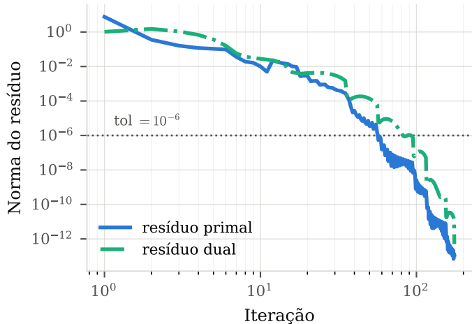
(b) Convergência do splitting (ADMM)
