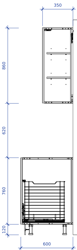
Corte A-A 1:25
