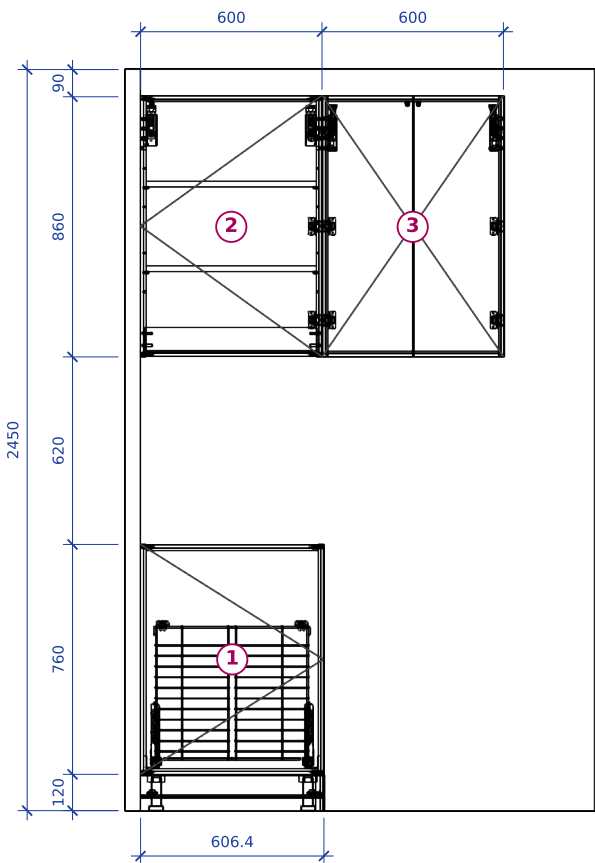
Alçado A1 1:25
