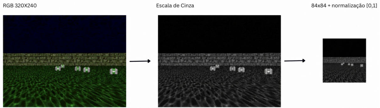
Figura 9 – Etapas de pré-processamento da observação visual do agente: imagem RGB original com resolução de 320 \times 240 pixels, conversão para escala de cinza, redimensionamento para 84 \times 84 pixels e normalização dos valores para o intervalo [0, 1] .
