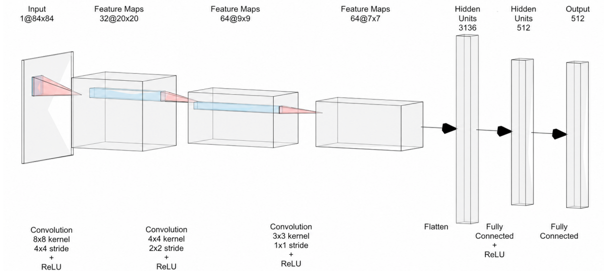
Figura 13 – Arquitetura compartilhada pelas redes alvo e preditora do RND, composta por três camadas convolucionais, uma etapa de vetorização e duas camadas totalmente conectadas.
