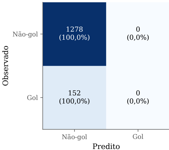
Limiar convencional (0,50)
