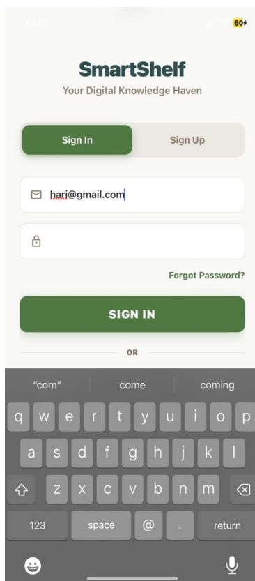
Figure 119 Unregister Login
