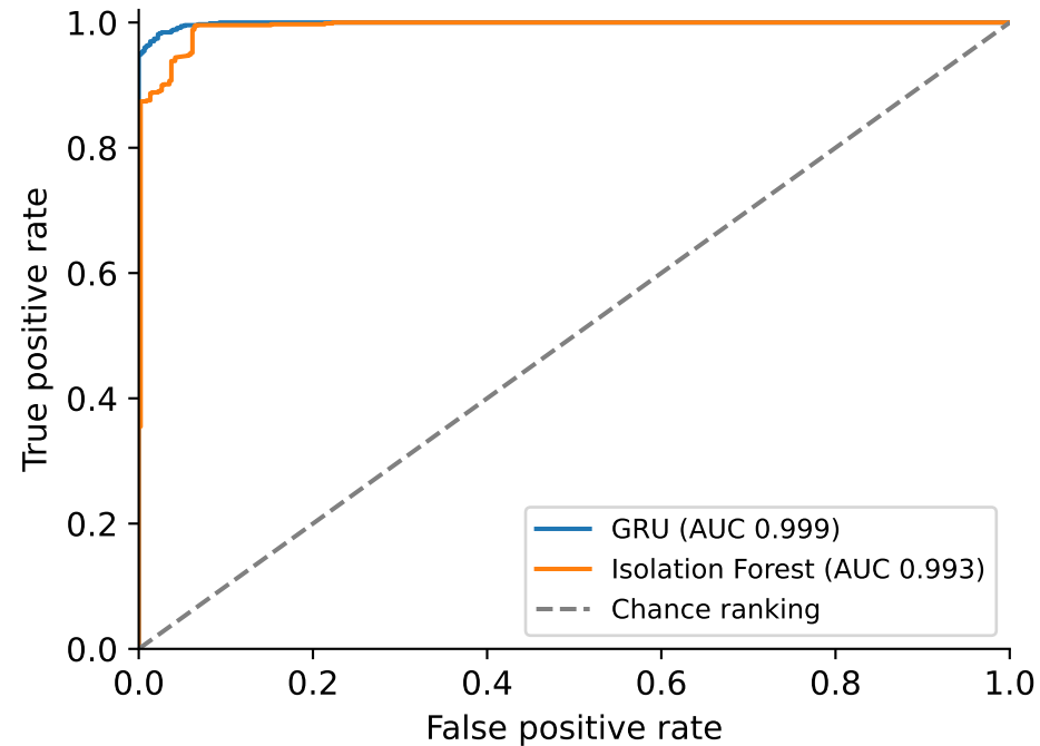
OB ROC
