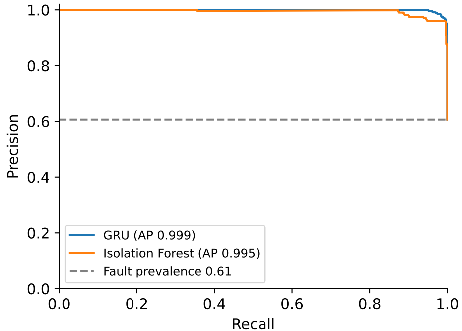
OB precision-recall
